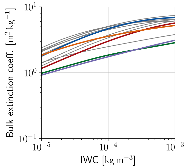
(d) Extinction (325 GHz)
