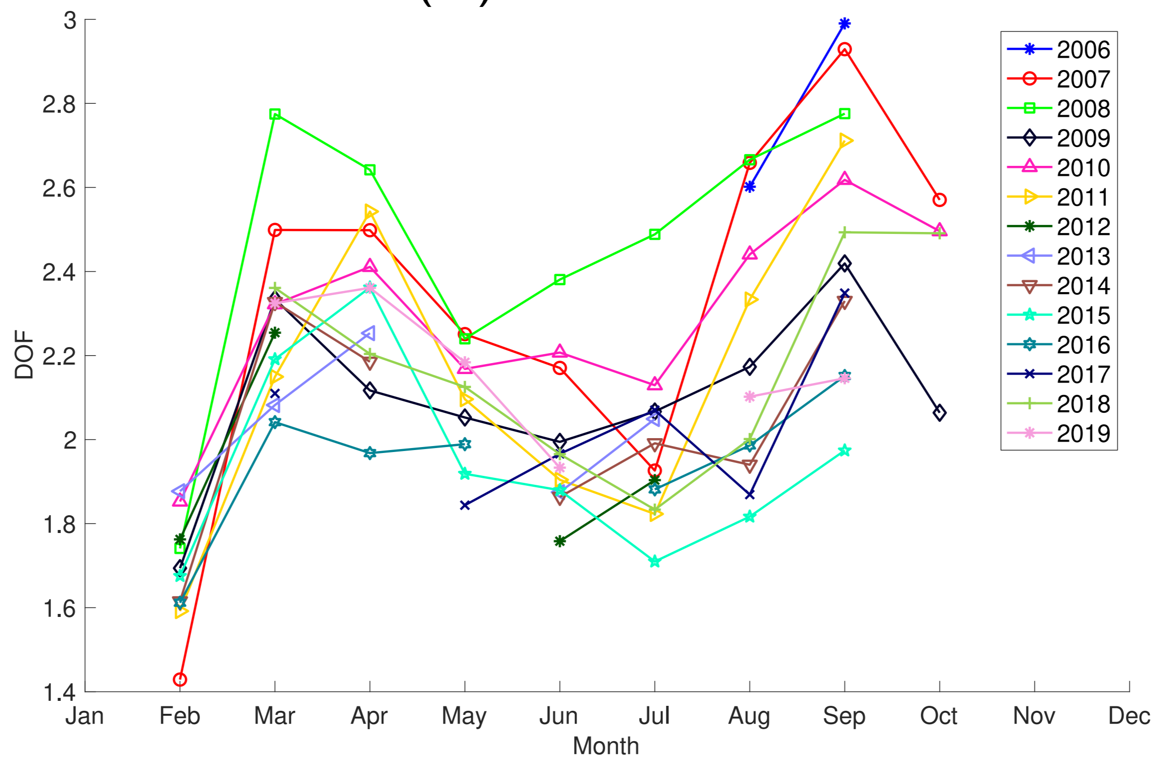
(d) NDACC
