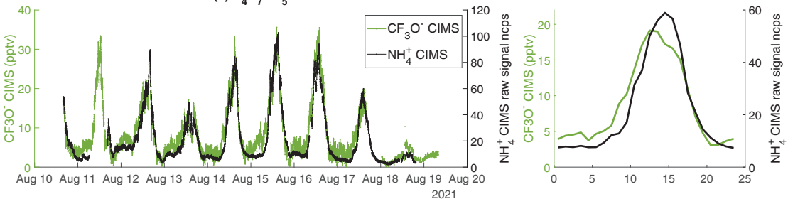
(b) C_5H_9NO_4
