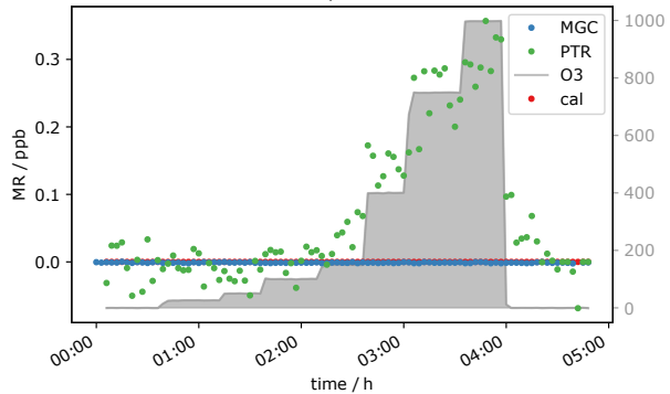
Isoprene
