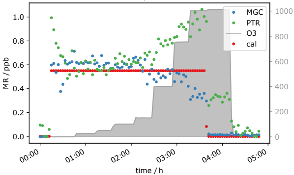
Isoprene
