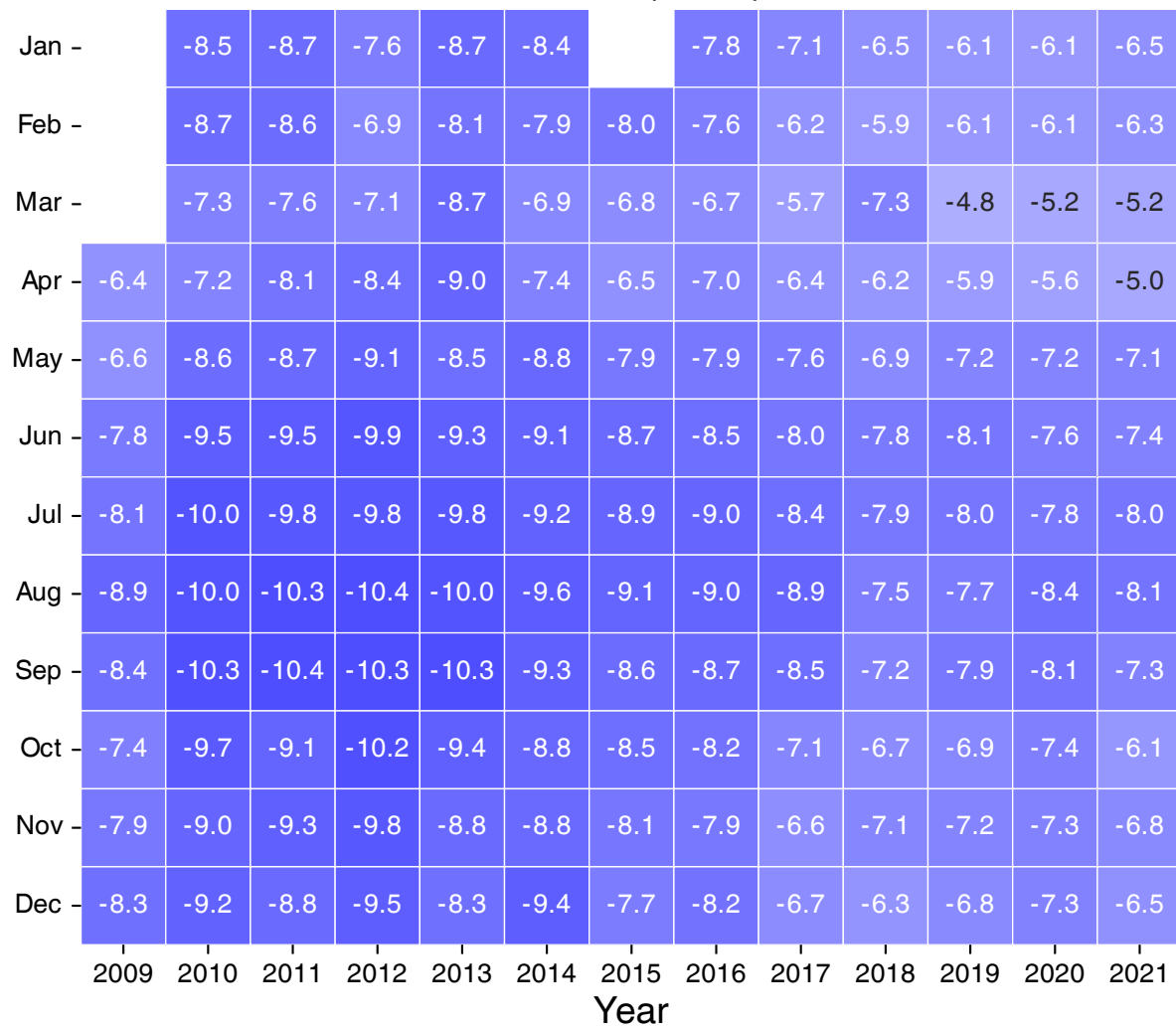
\Delta XCH_4 (Land)
