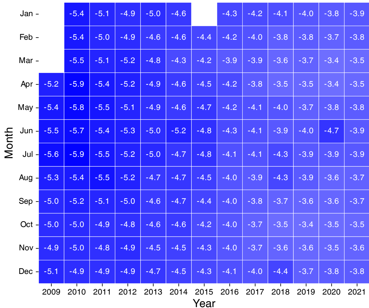
\Delta XCO_2 (Ocean)
