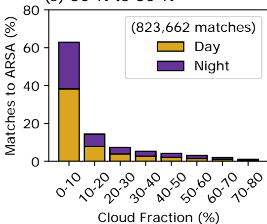
(e) 30°N to 60°N
