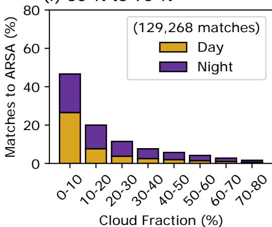
(f) 60°N to 90°N
