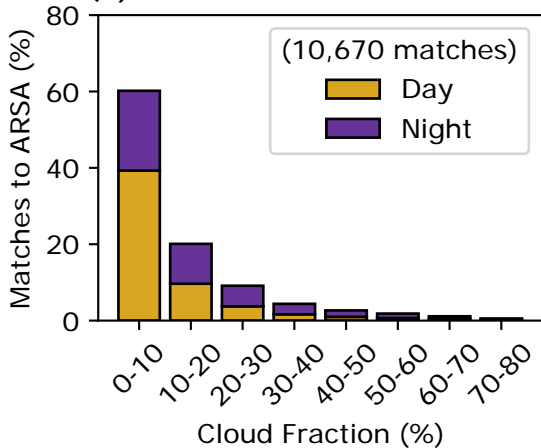
(d) 30°S to 30°N
