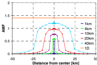
AMF 313 nm
