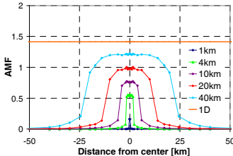
AMF 313 nm
