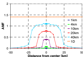
AMF 313 nm
