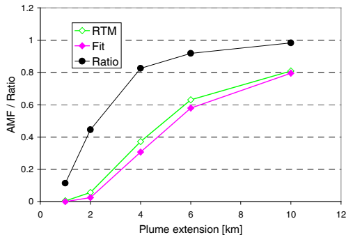
(d) 313 nm, 4 \cdot 10^{30} molecules
