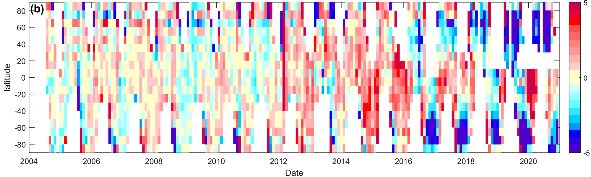
OSIRIS v7 minus MLS 40 km
