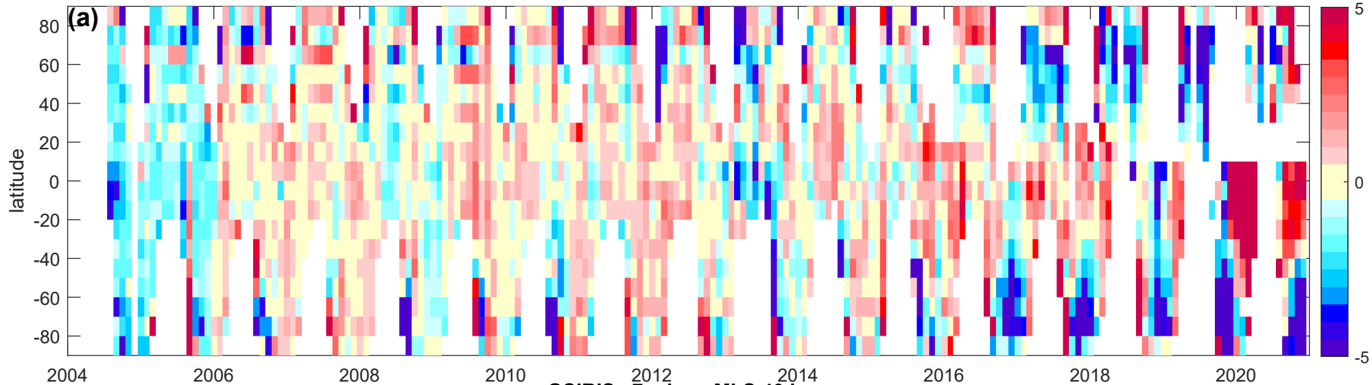
OSIRIS v7 minus MLS 40 km
