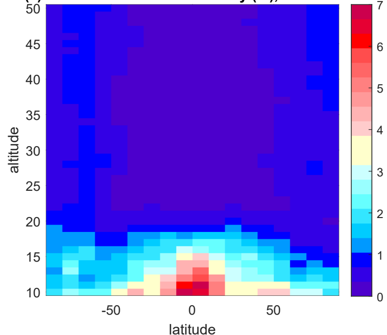
(d) SAGE-CCI-OMPS uncertainty (%), 2015-2020
