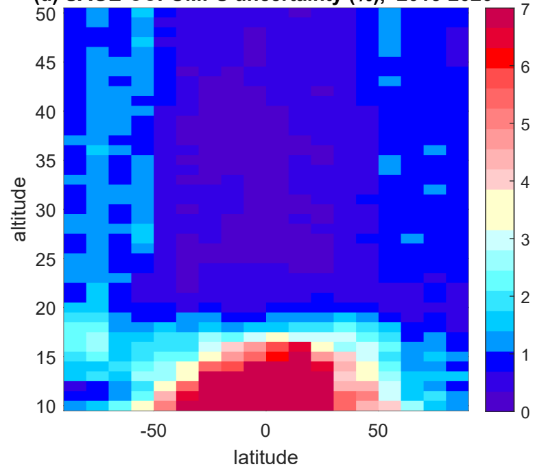
(d) SAGE-CCI-OMPS uncertainty (%), 2015-2020
