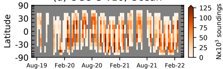
(d) OCO-3 v10, Ocean
