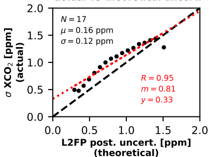
(d) OCO-3 v10, land-nadir actual vs theoretical uncert.
