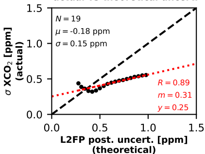
(d) OCO-3 v10, ocean-glint actual vs theoretical uncert.
