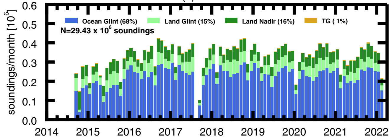
(a) OCO-2 v10
