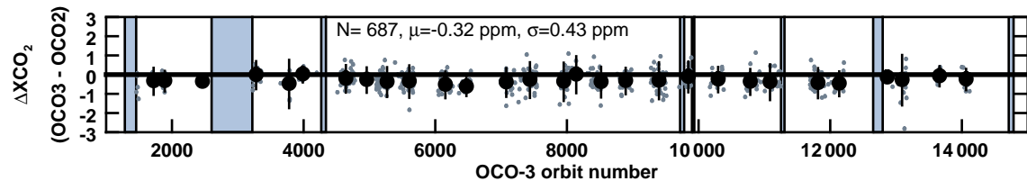
(d) v10 \Delta XCO_2 after ad hoc correction
