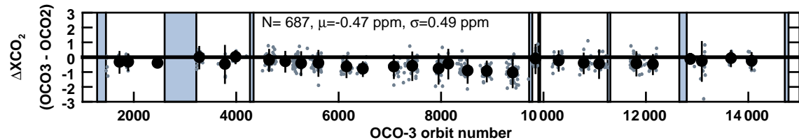
(b) v10 \Delta XCO_2 vs OCO-3 WCO_2 ZLO
