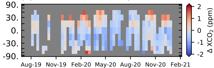
(d) OCO-3 v10 with adhoc, Ocean-Glint
