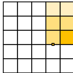
(f) ■ Isoborneol
