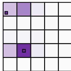
(d) ■ Decane
