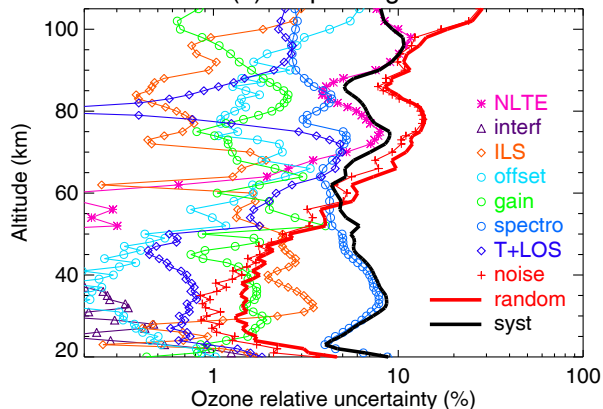
(d) Northern midlatitude spring night MA
