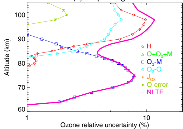
(d) Northern midlatitude spring night MA
