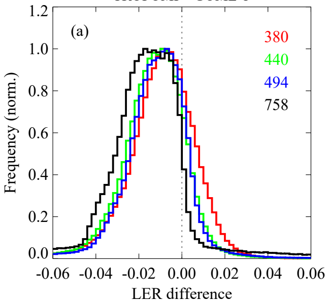
TROPOMI - SCIAMACHY
