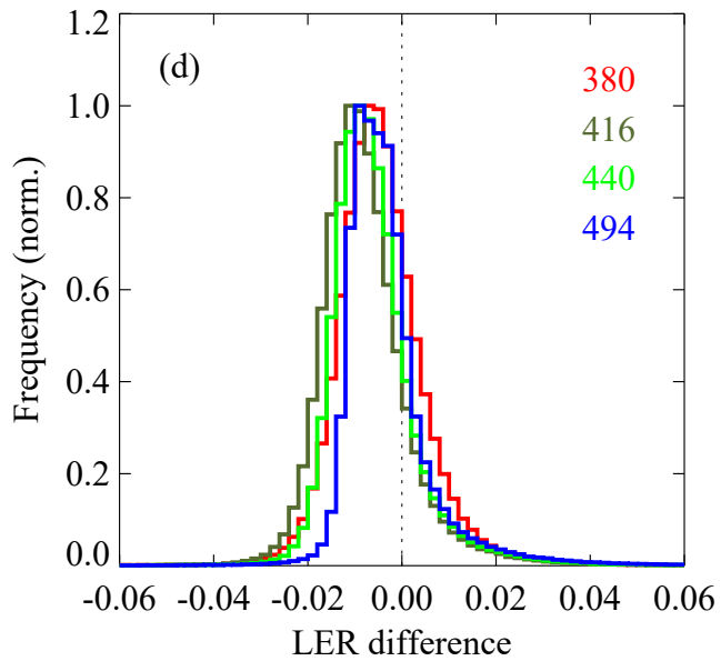
TROPOMI - OMI
