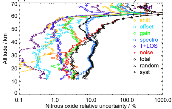
(d) Northern midlatitude summer day RR
