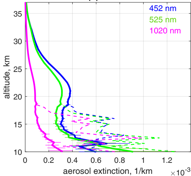
(e) SAGE II
