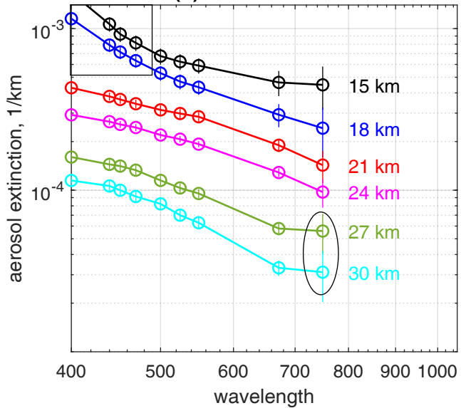
(d) FMI-GOMOSaero
