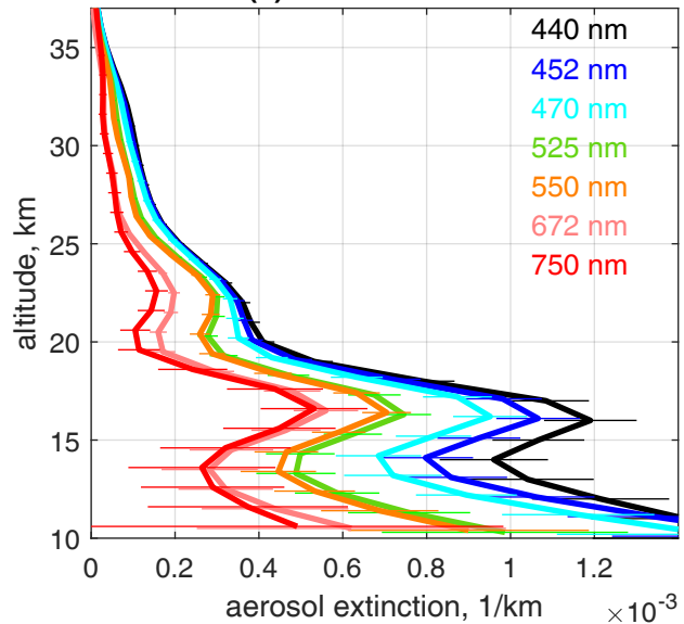
(d) FMI-GOMOSaero
