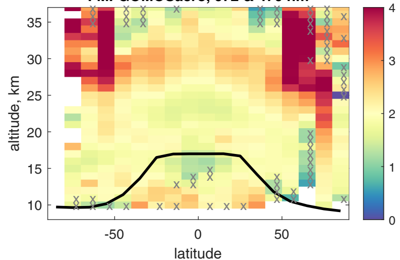
FMI-GOMOSaero, 672 & 470 nm
