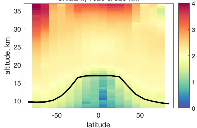
SAGE II, 1020 & 525 nm
