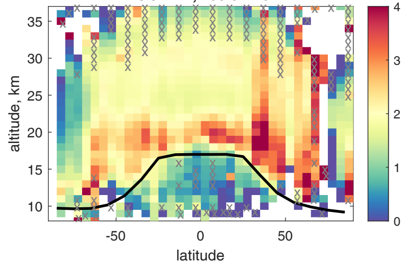
AERGOM v4, 750 & 470 nm
