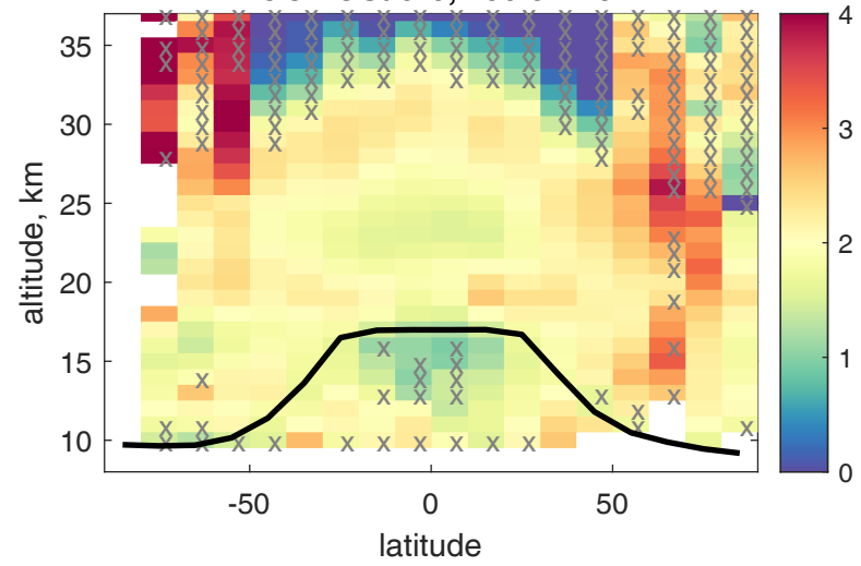
FMI-GOMOSaero, 750 & 470 nm
