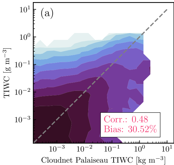
CPCIR
