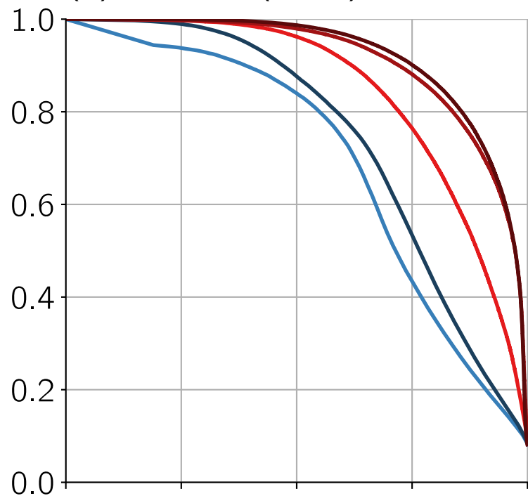
(d) MRMS (2021)
