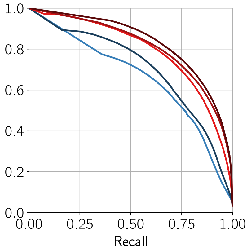
(d) MRMS (2021)
