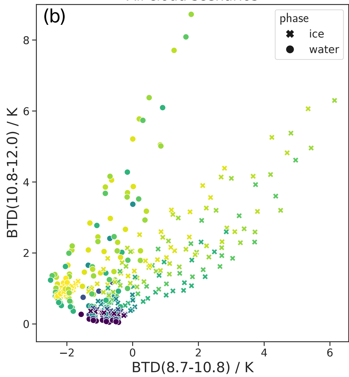
All cloud scenarios
