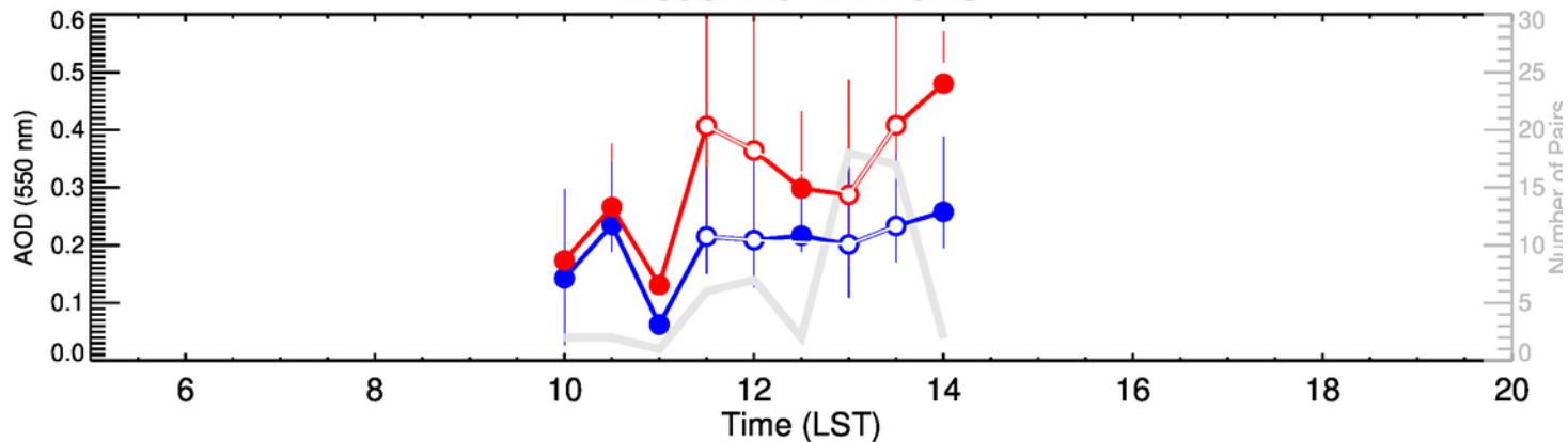
Medenine-IRA-OND
