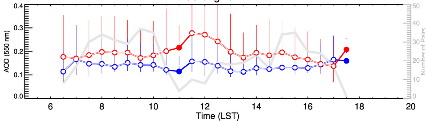
Sorong-JFM
