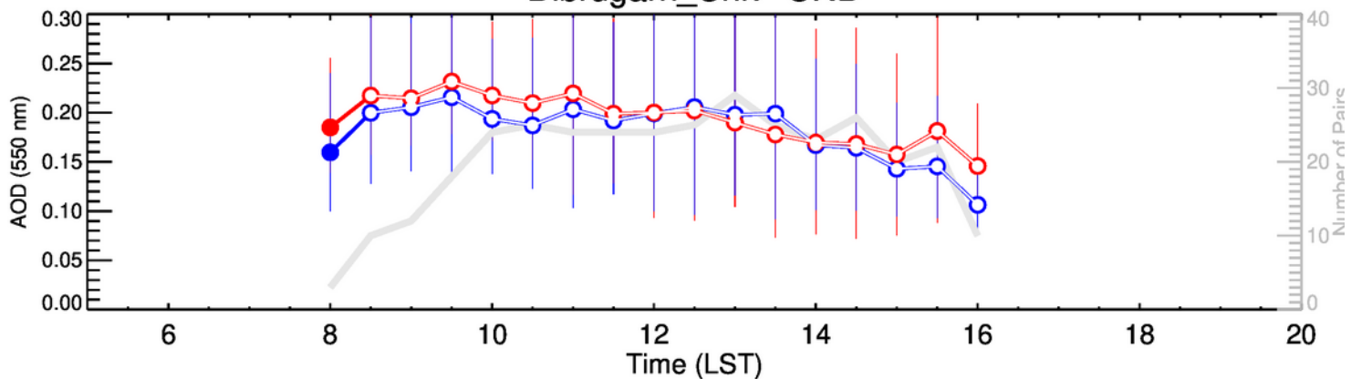
Dibrugarh_ Univ-JFM
