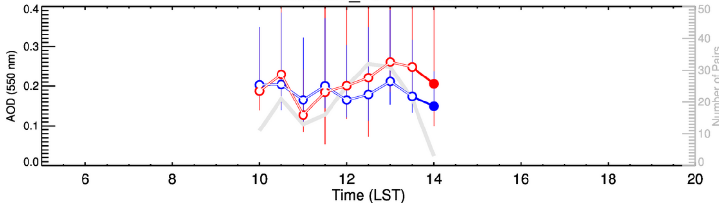
Lamezia_Terme-OND
