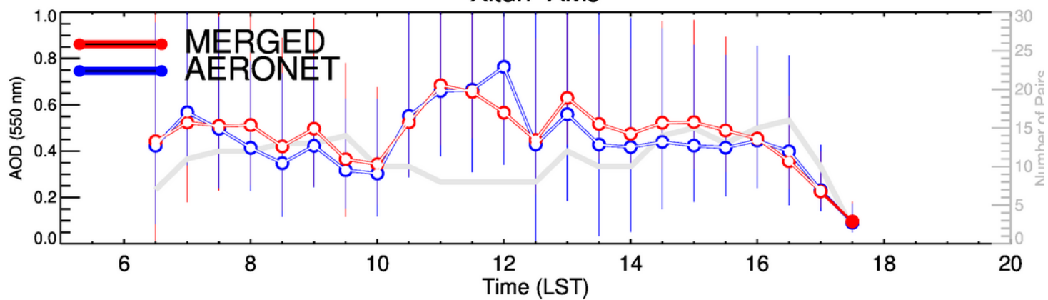
Xitun-JAS
