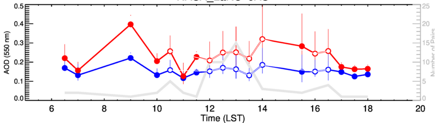
NASA_LaRC-OND
