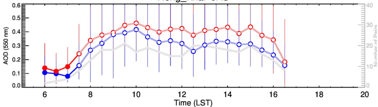
Nong_Khai-OND
