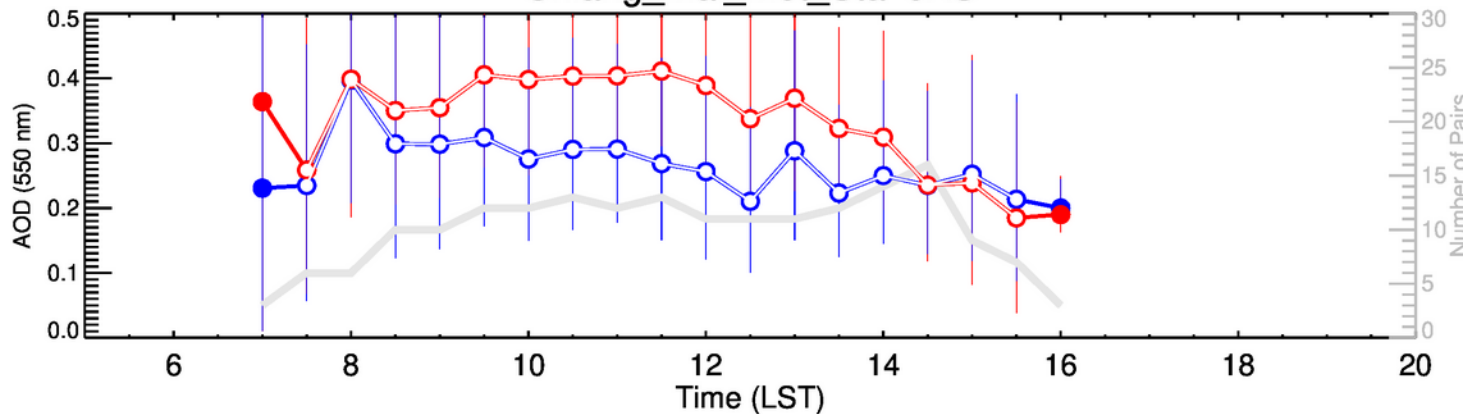
Chiang_Mai_Met_Sta-OND
