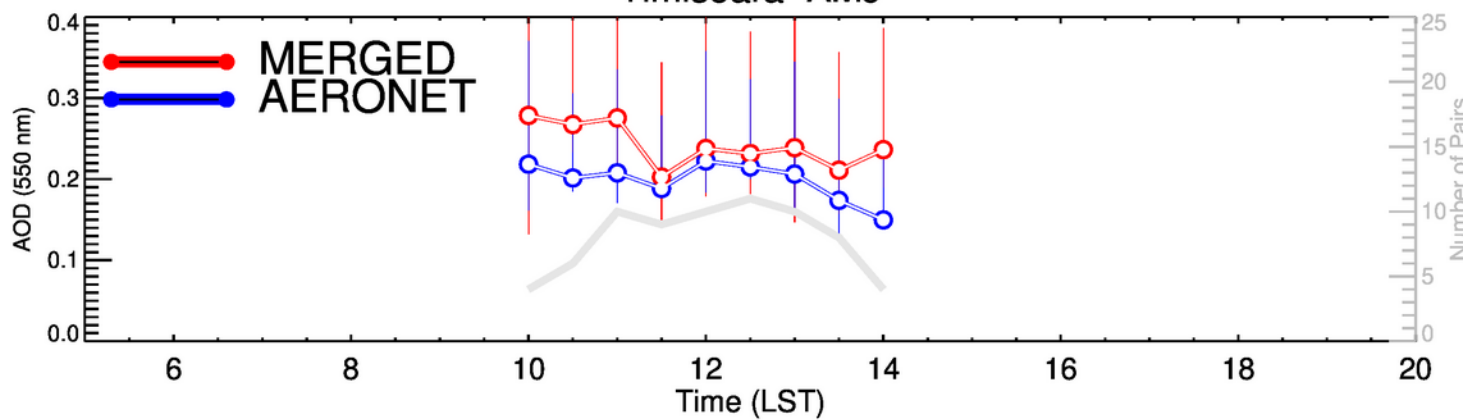
Timisoara-JAS
