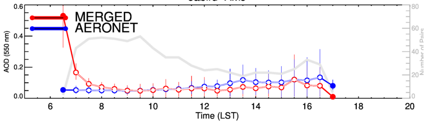
Jabiru-JAS
