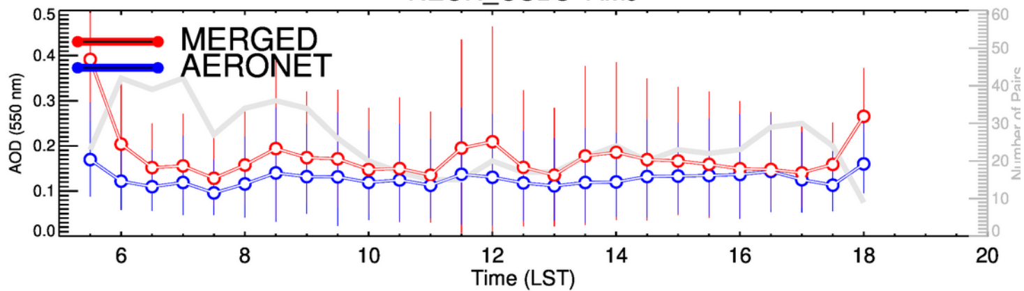
NEON_OSBS-JAS
