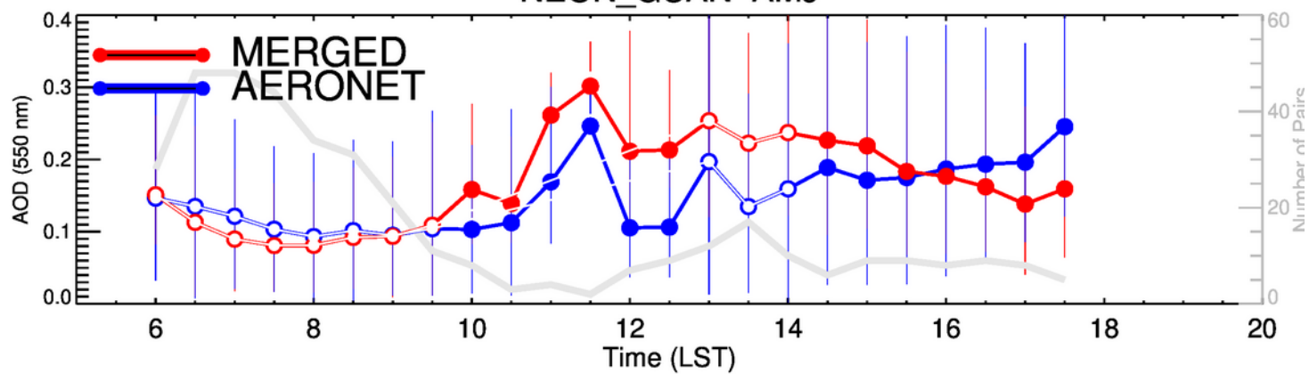
NEON_GUAN-JAS
