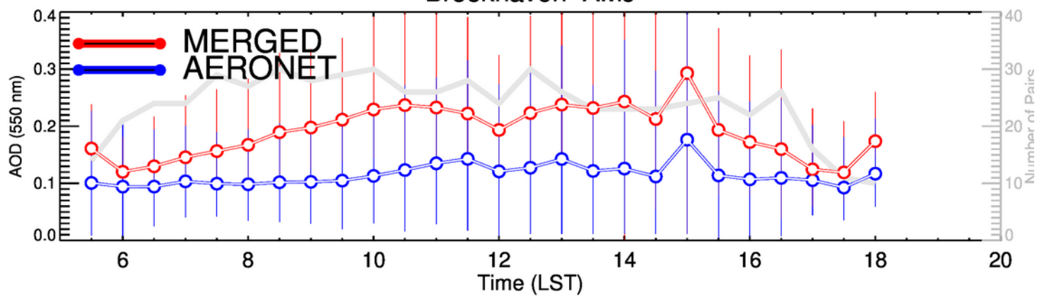
Brookhaven-JAS
