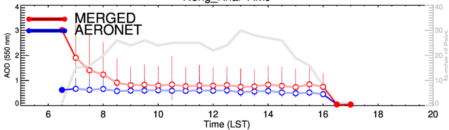
Nong_Khai-JAS
