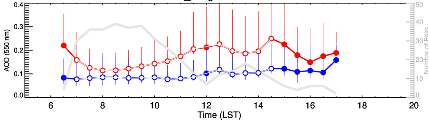
La_Parguera-JFM
