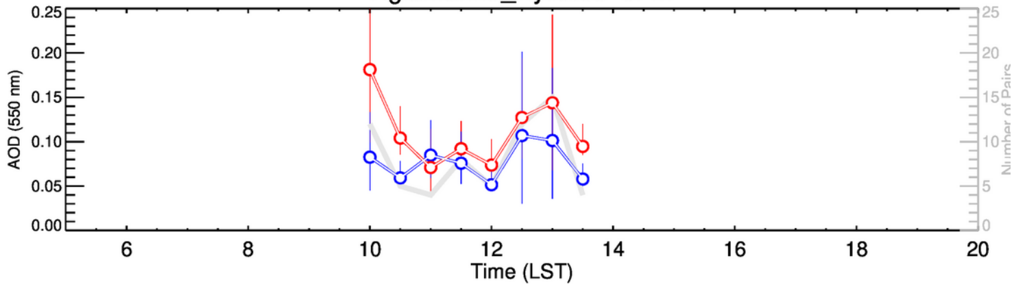
AgiaMarina_Xyliatou-JFM
