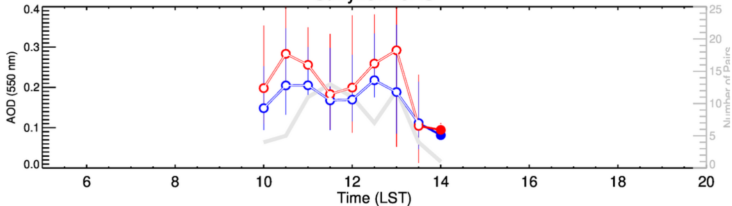
Strzyzow-OND
