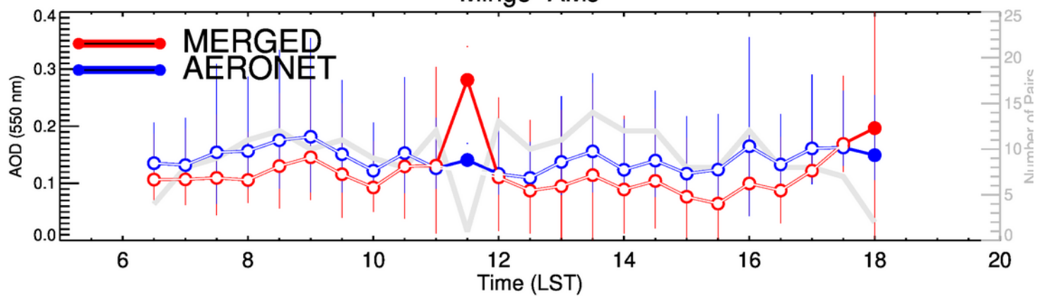
Mingo-JAS
