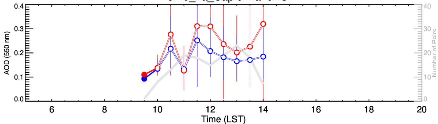
Rome_La_Sapienza-OND
