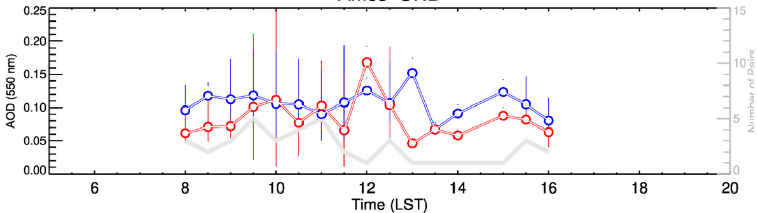
Ames-JFM
