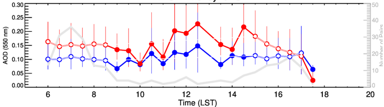
NEON-Disney-OND
