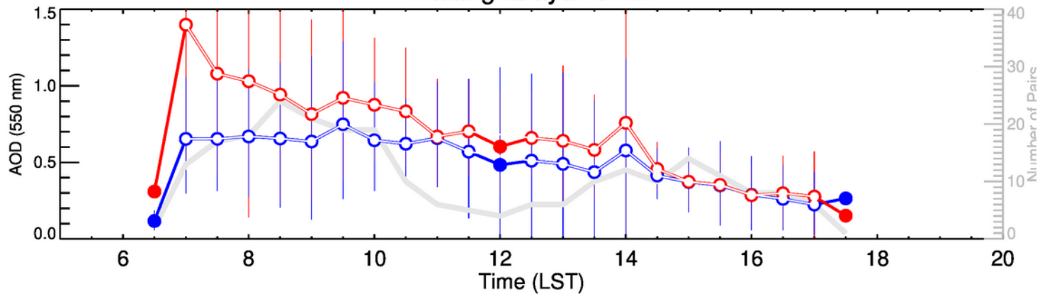
Palangkaraya-JFM
