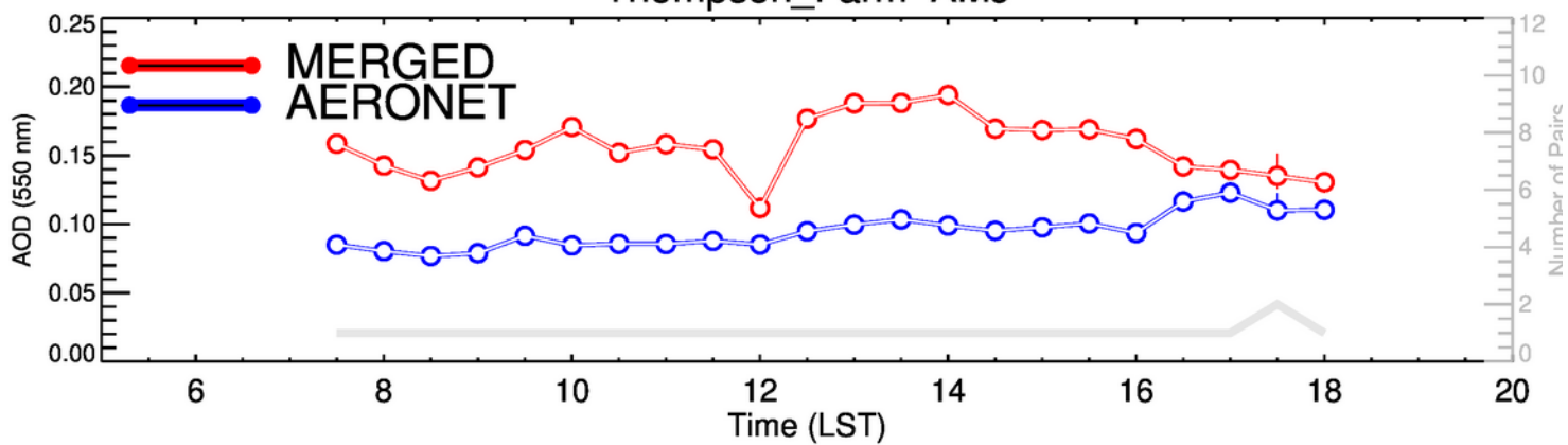
Thompson_Farm-JAS
