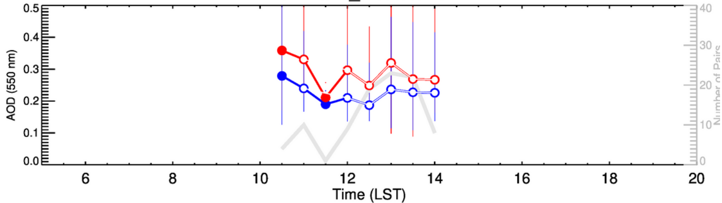
Weizmann_Institute-JFM
