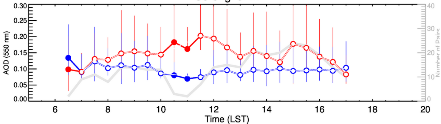
Sorong-JFM
