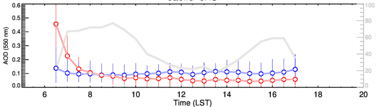
Jabiru-OND
