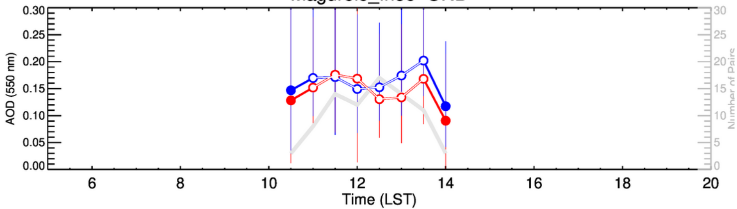
Magurele_Inoe-JFM
