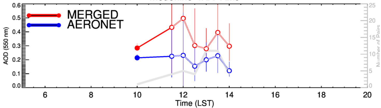
Medenine-IRA-JAS
