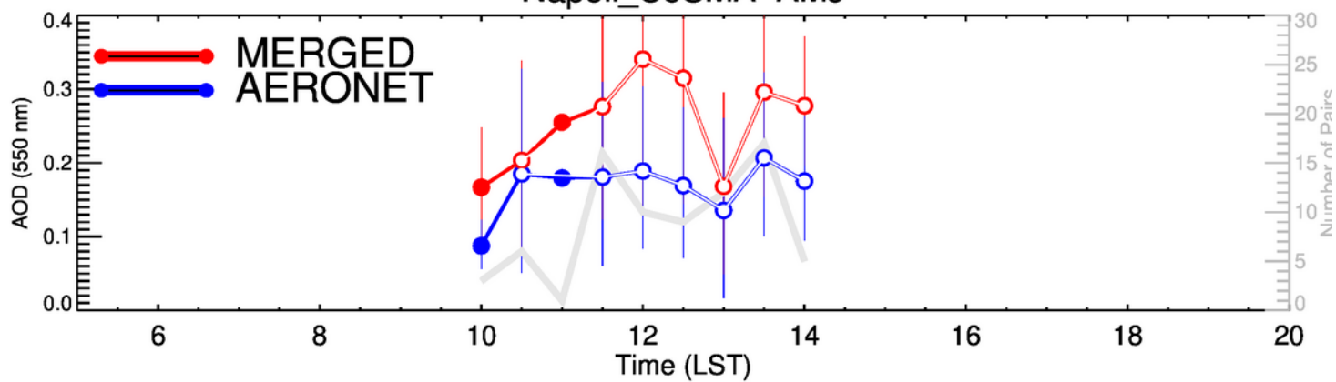
Napoli_CeSMA-JAS
