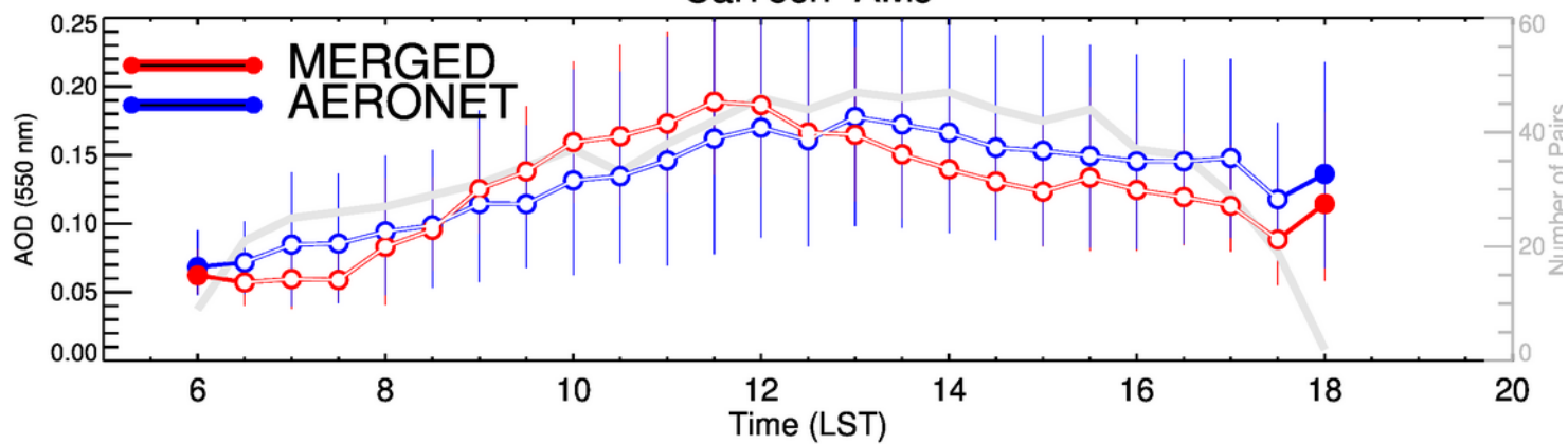
CalTech-JAS
