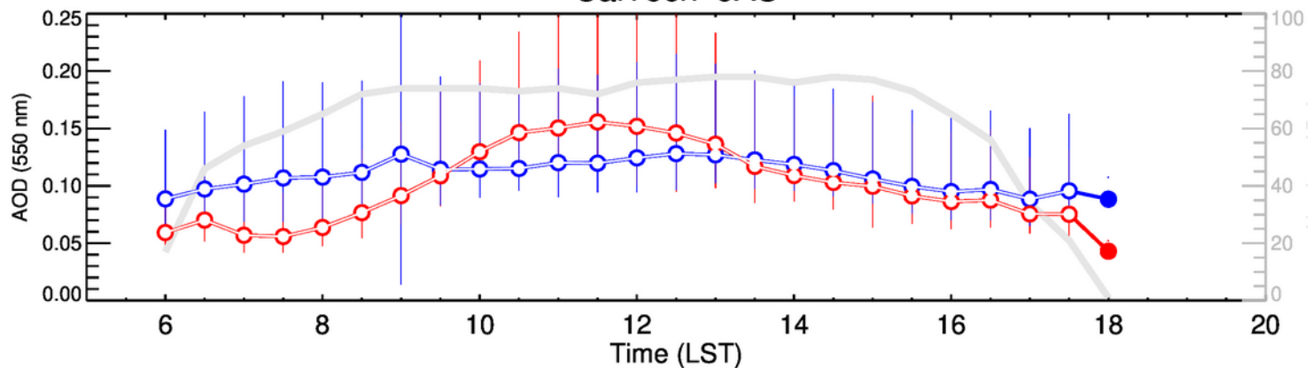
CalTech-OND
