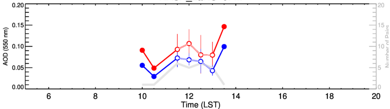
NASA_LaRC-JFM
