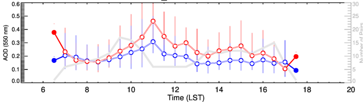
Alta_Floresta-JFM
