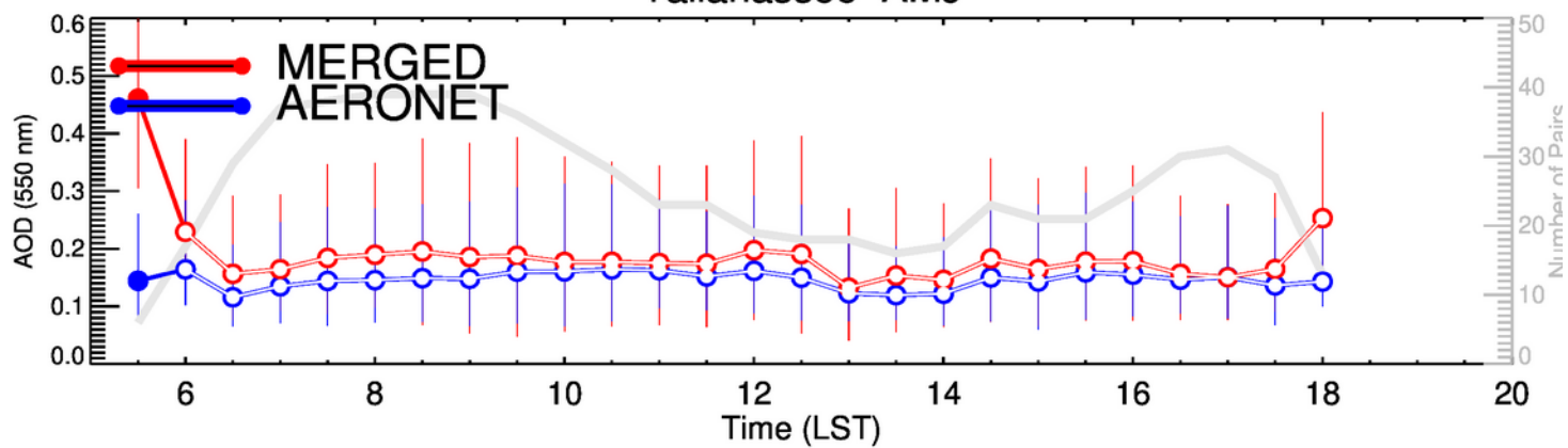
Tallahassee-JAS
