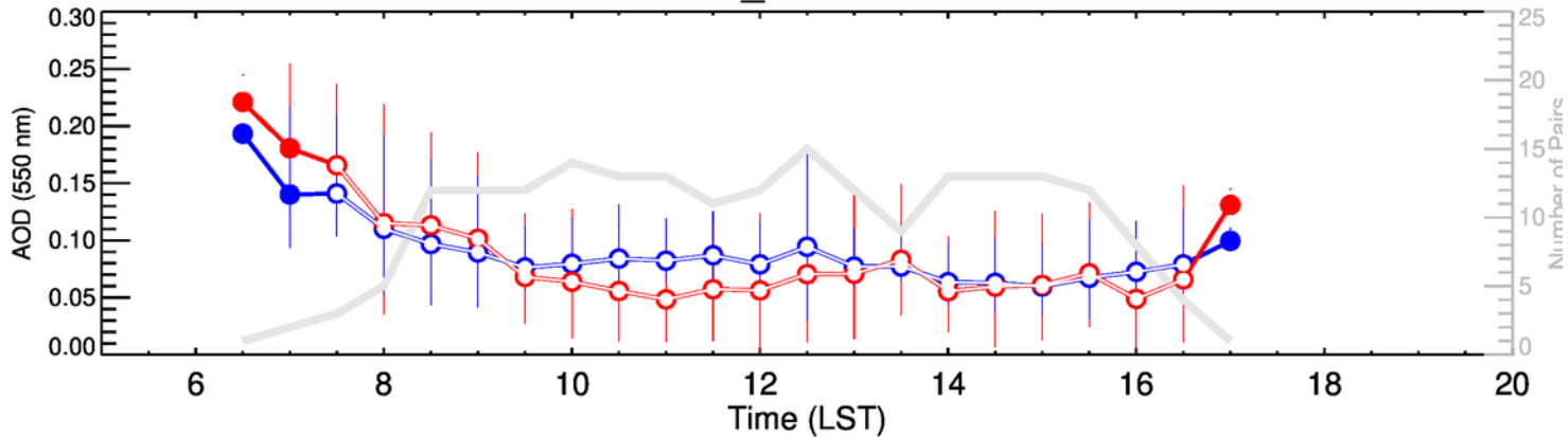
NEON_ORNL-JFM
