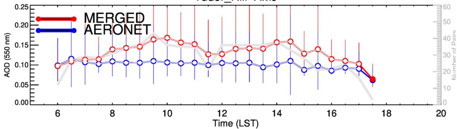
Tudor_Hill-JAS
