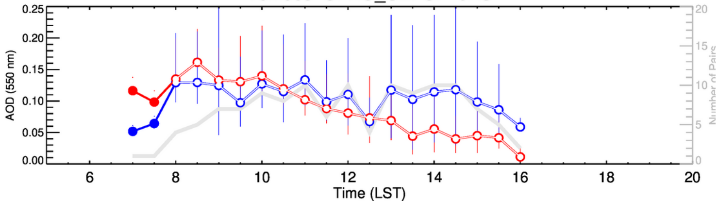
Temuco-UFRO_CEFOP-OND
