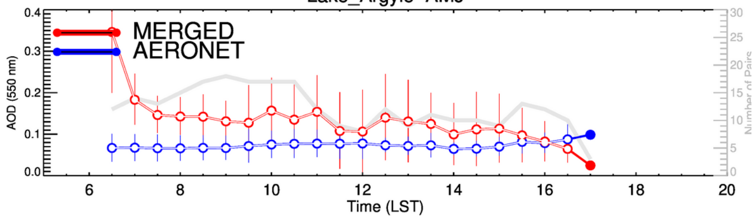
Lake_Argyle-JAS
