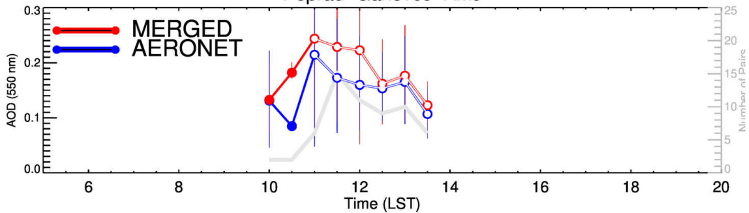
Poprad-Ganovce-JAS
