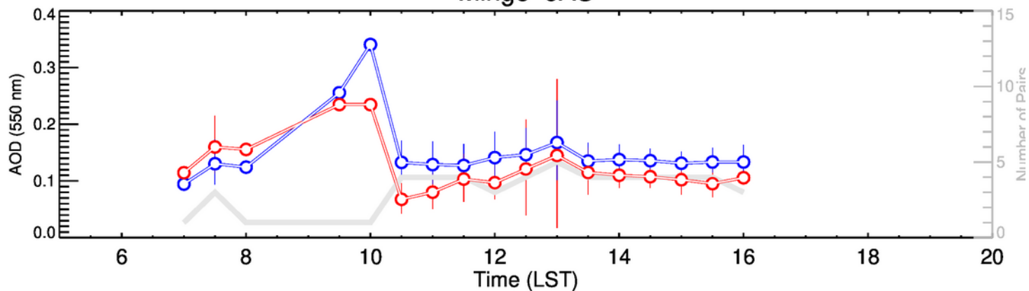
Mingo-OND
