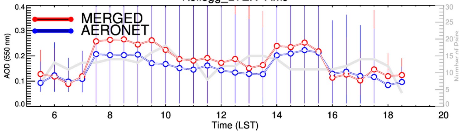
Kellogg_LTER-JAS
