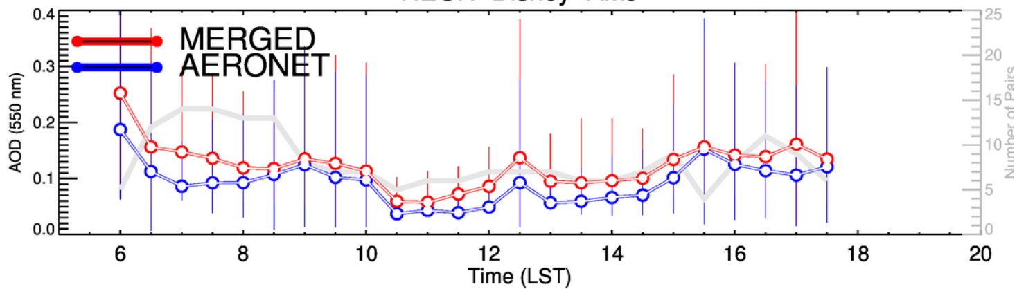
NEON-Disney-JAS
