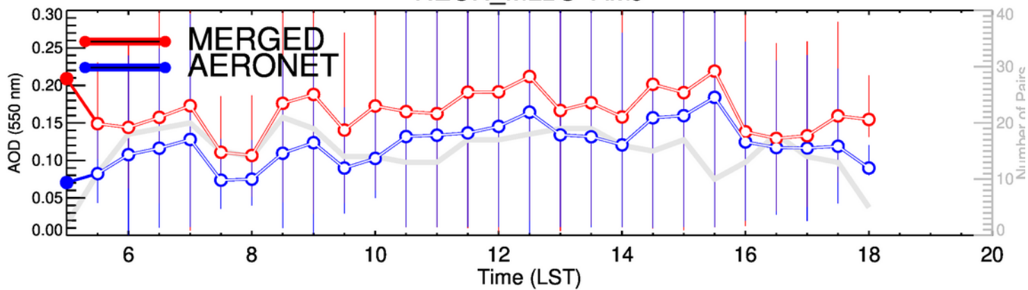
NEON_MLBS-JAS
