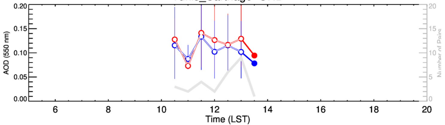
Tunis_Carthage-JFM
