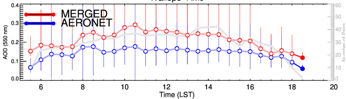
Wallops-JAS
