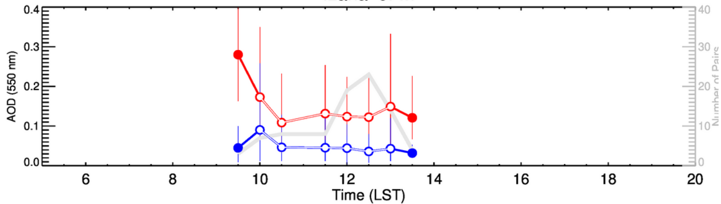
Izana-JFM
