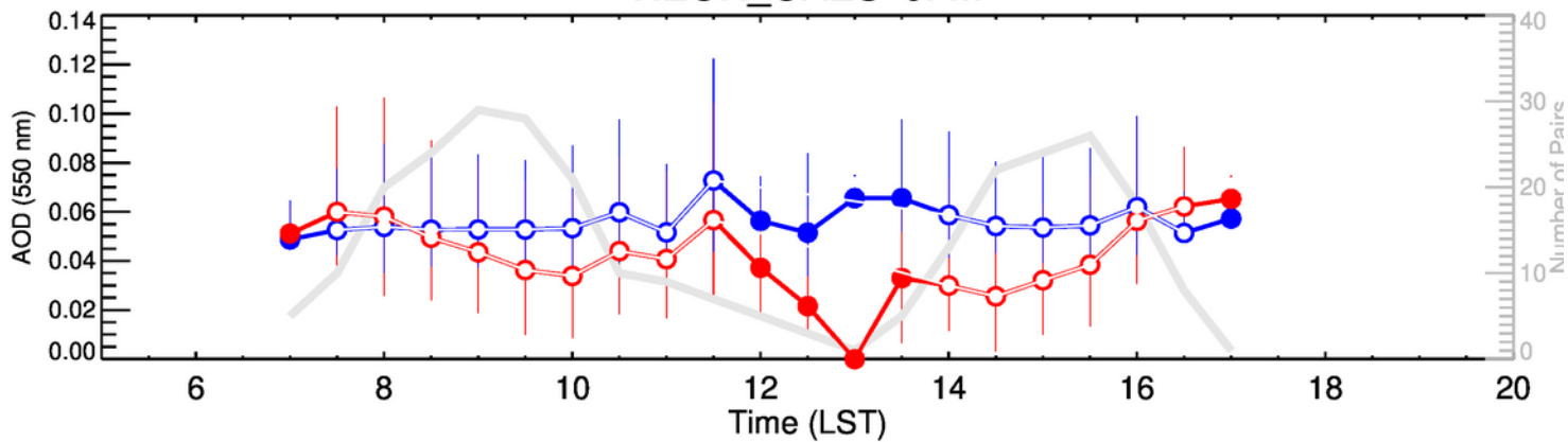
NEON_OAES-JFM
