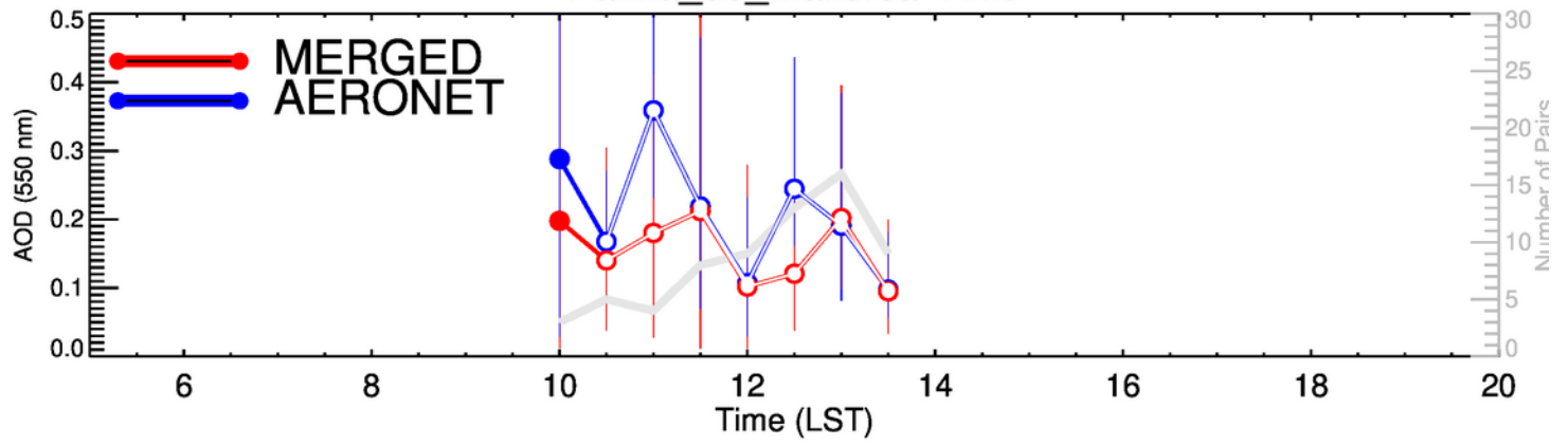
Palma_de_Mallorca-JAS
