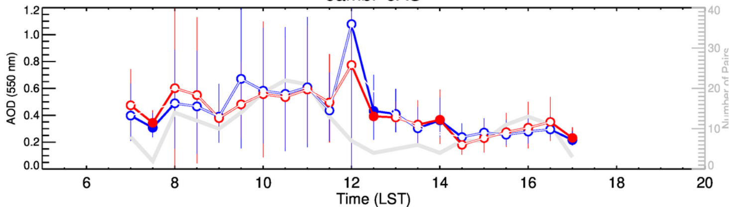
Jambi-OND
