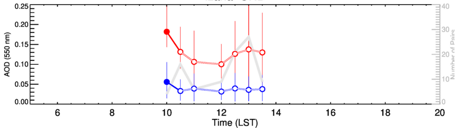
Izana-JFM
