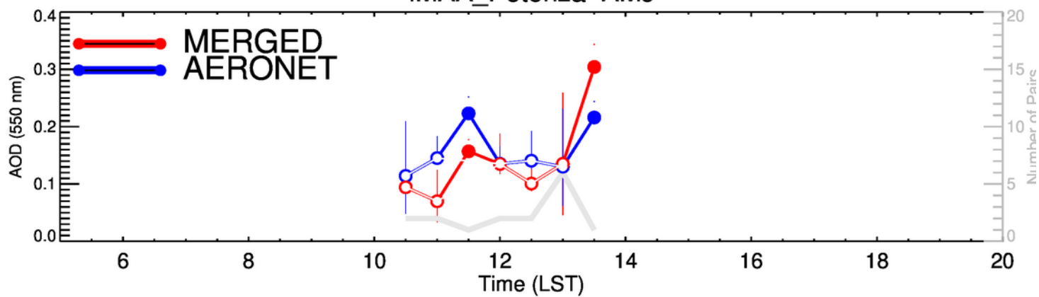
IMAA_Potenza-JAS
