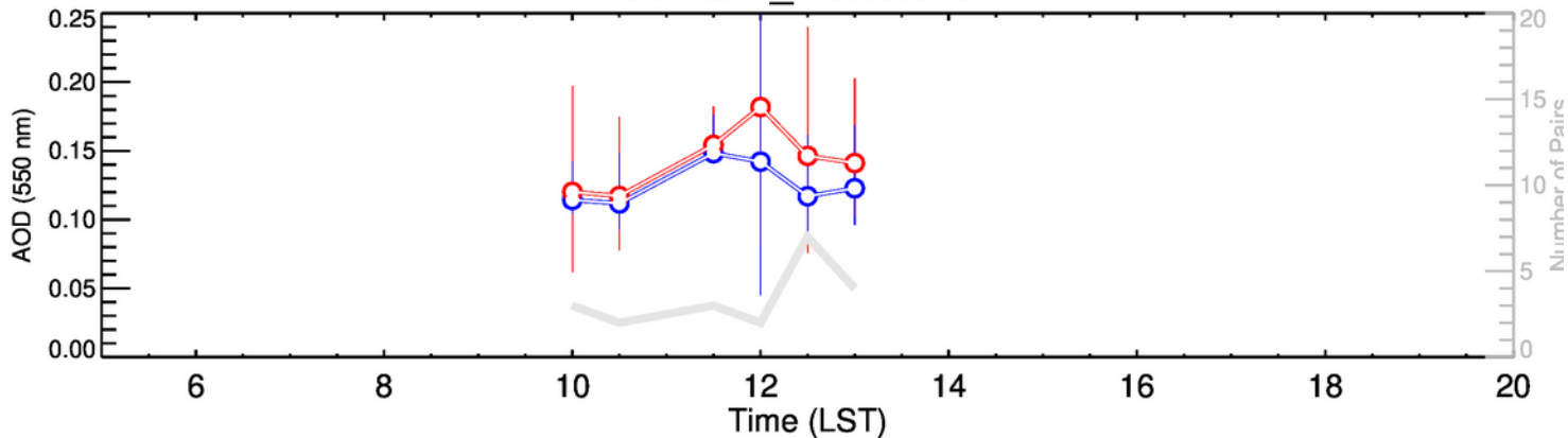
Weizmann_Institute-JFM
