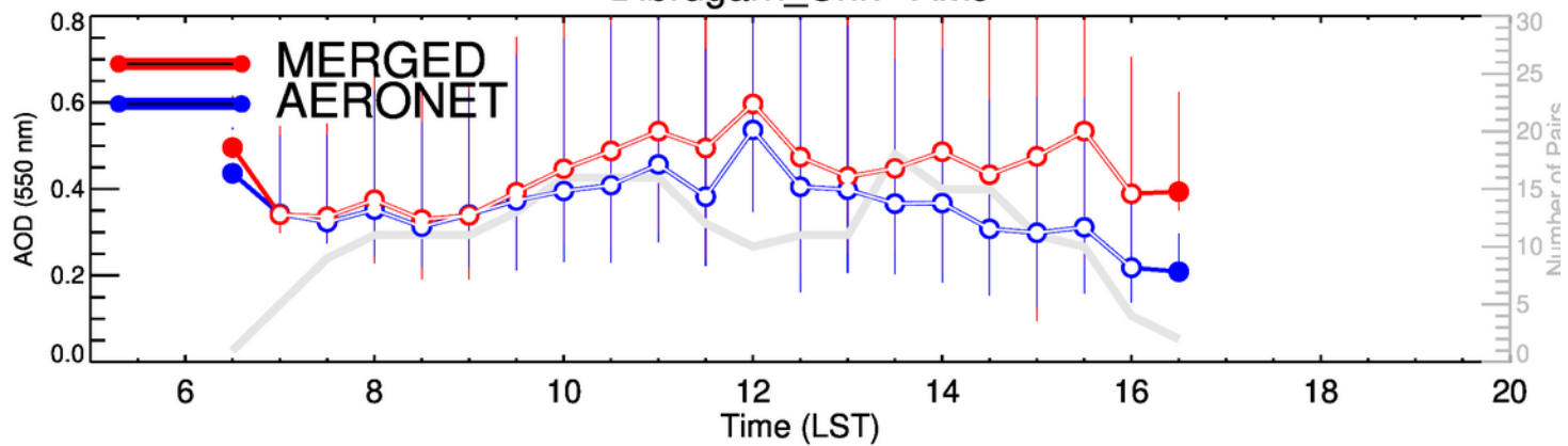
Dibrugarh_ Univ-OND
