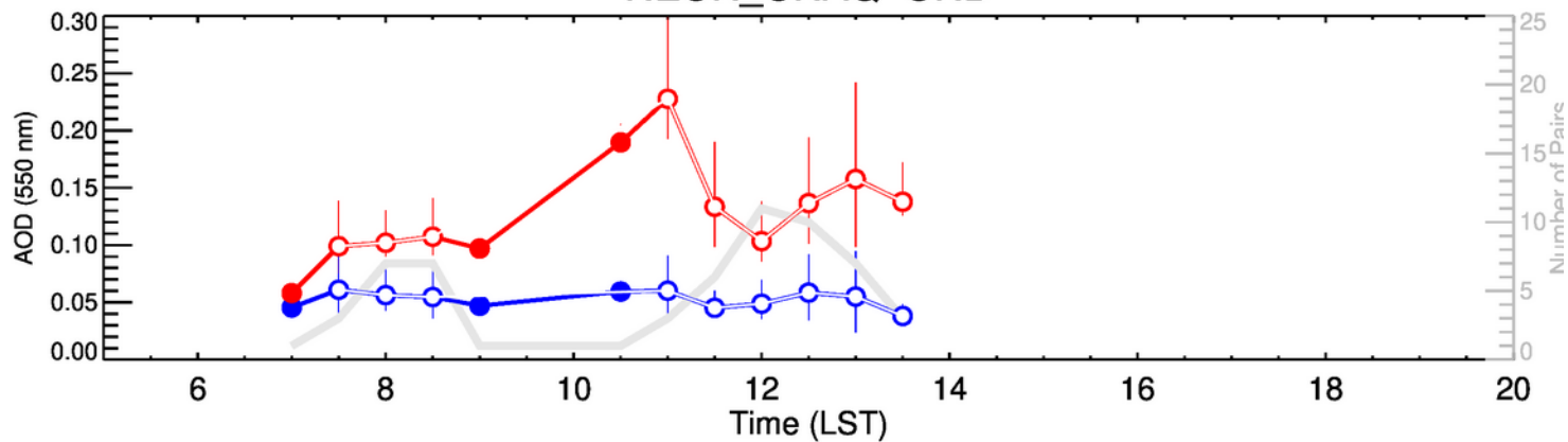
NEON_ONAQ-JFM
