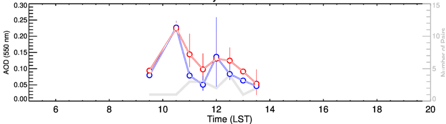
Strzyzow-JFM
