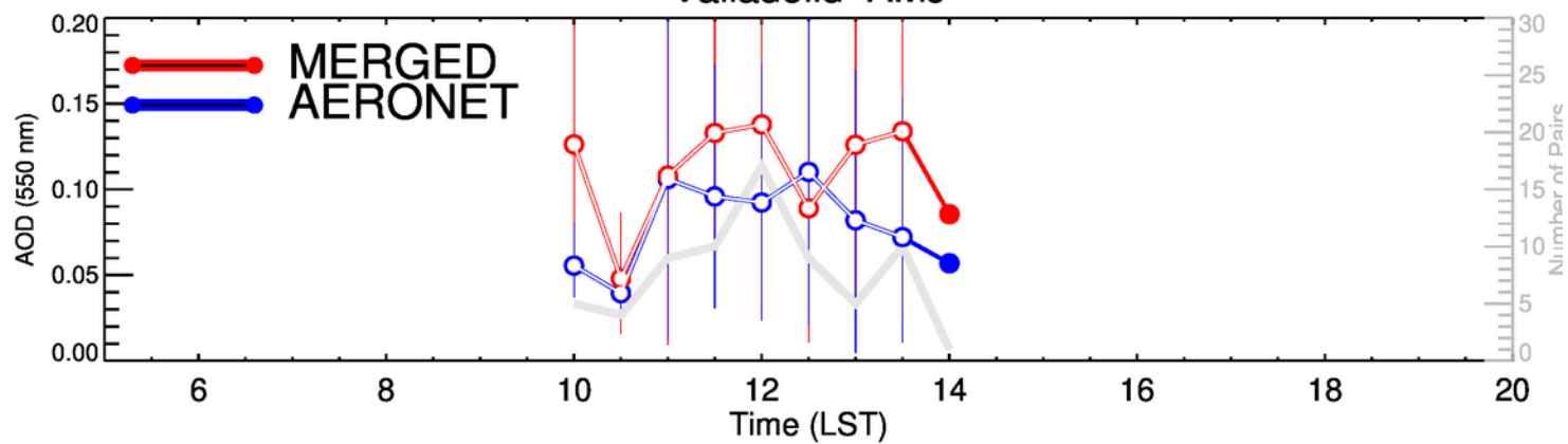
Valladolid-OND
