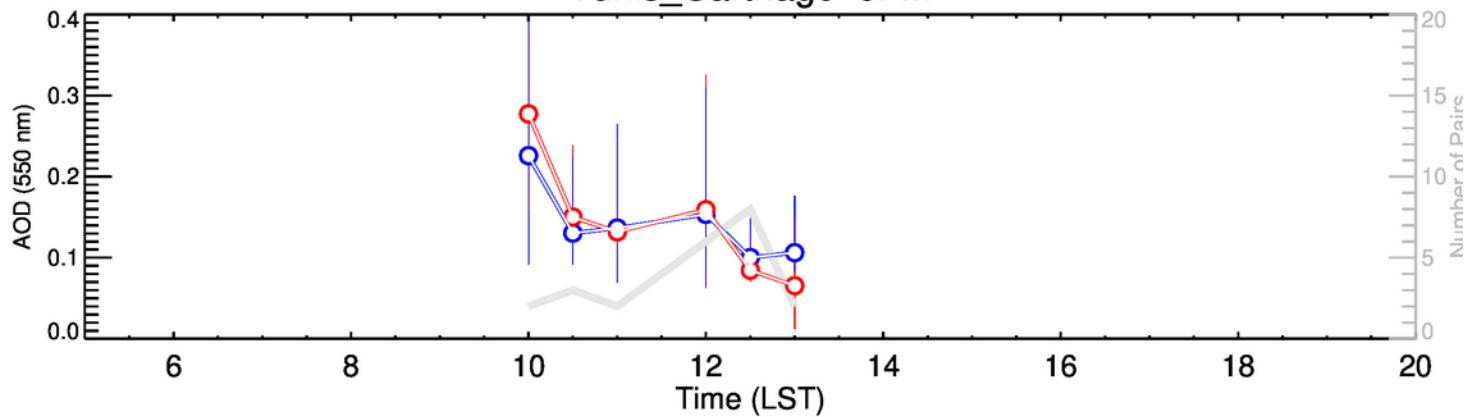
Tunis_Carthage-JFM
