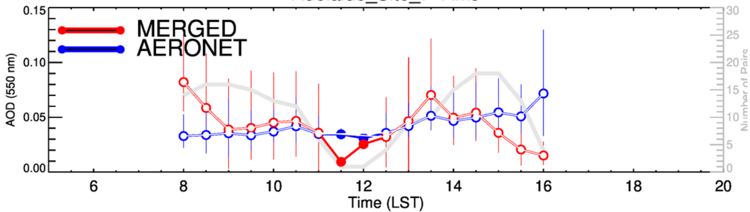
Adelaide_Site_7-JAS
