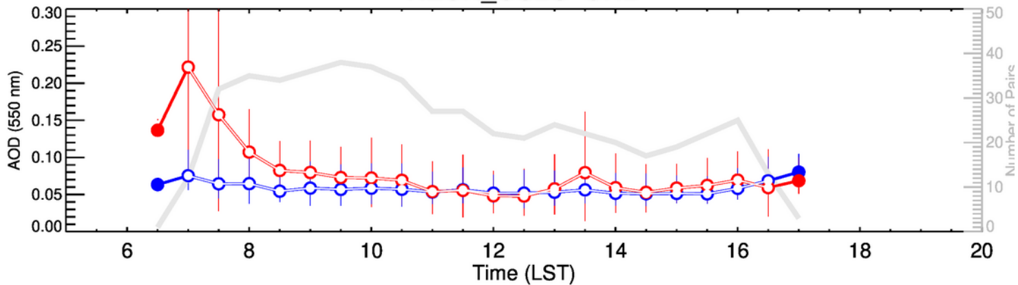
NEON_OSBS-JFM
