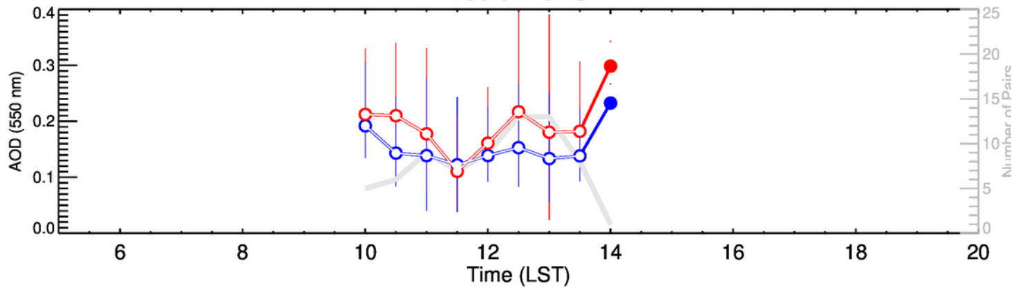
Toulon-OND
