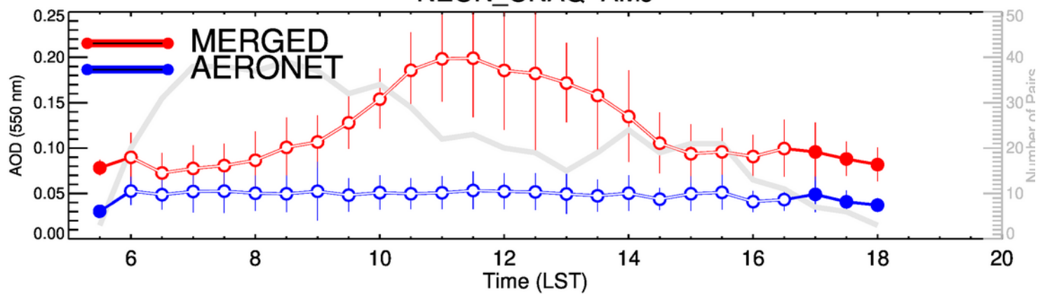
NEON_ONAQ-JAS
