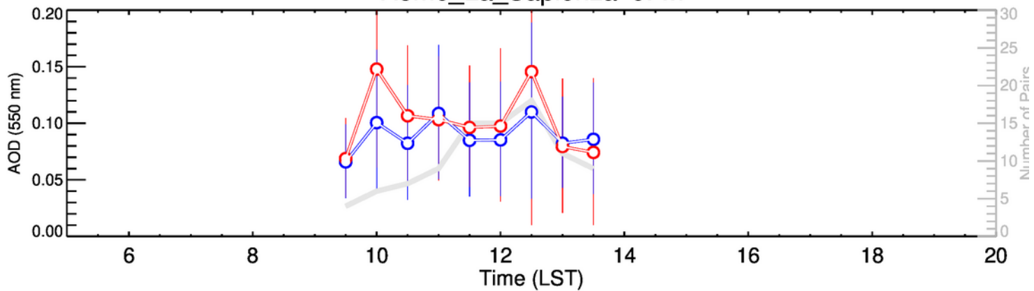
Rome_La_Sapienza-JFM
