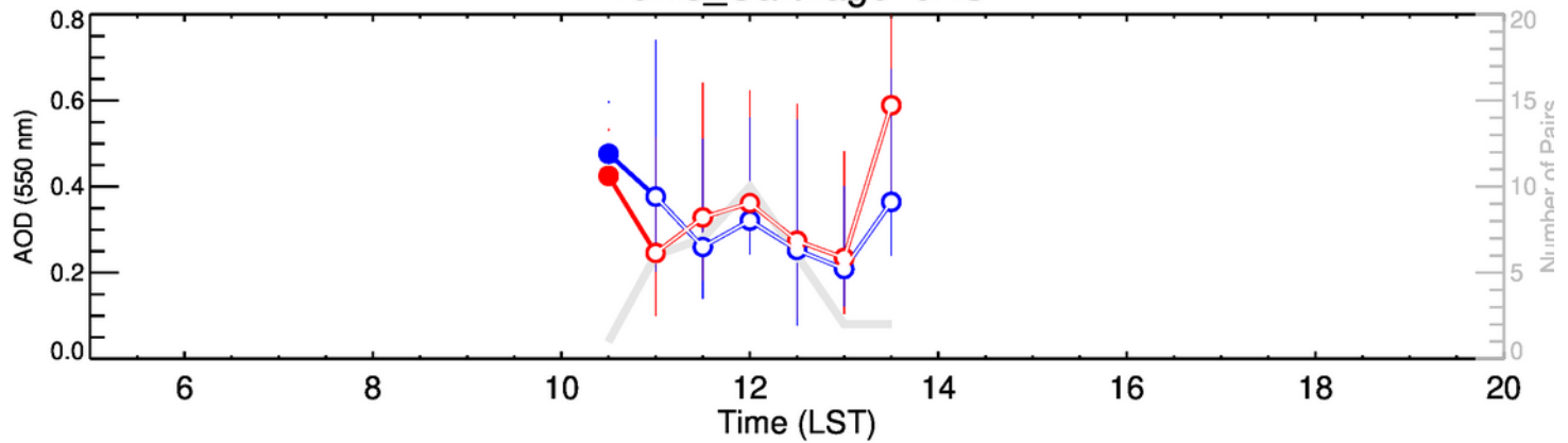
Tunis_Carthage-OND
