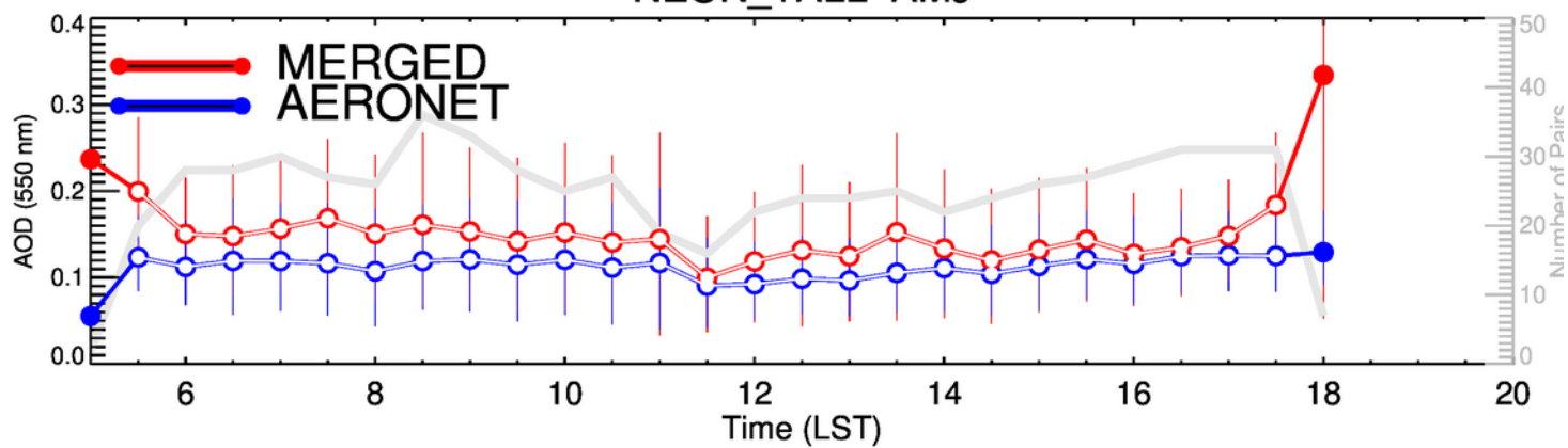
NEON_TALL-JAS
