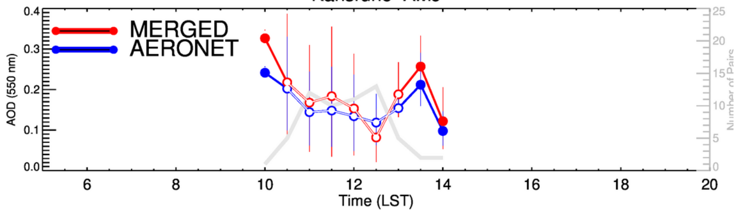
Karlsruhe-JAS
