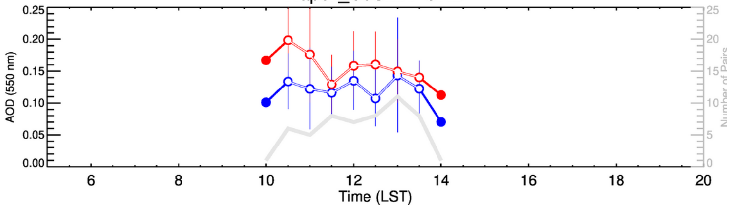
Napoli_CeSMA-JFM
