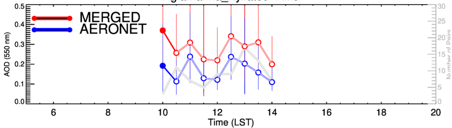
AgiaMarina_Xyliatou-JAS
