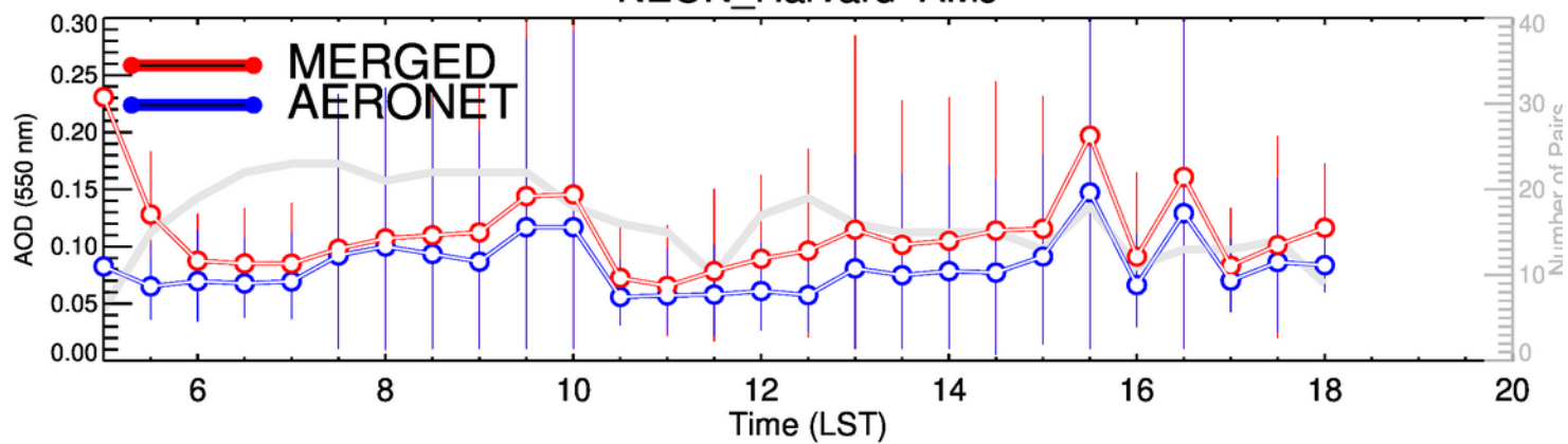
NEON_Harvard-JAS
