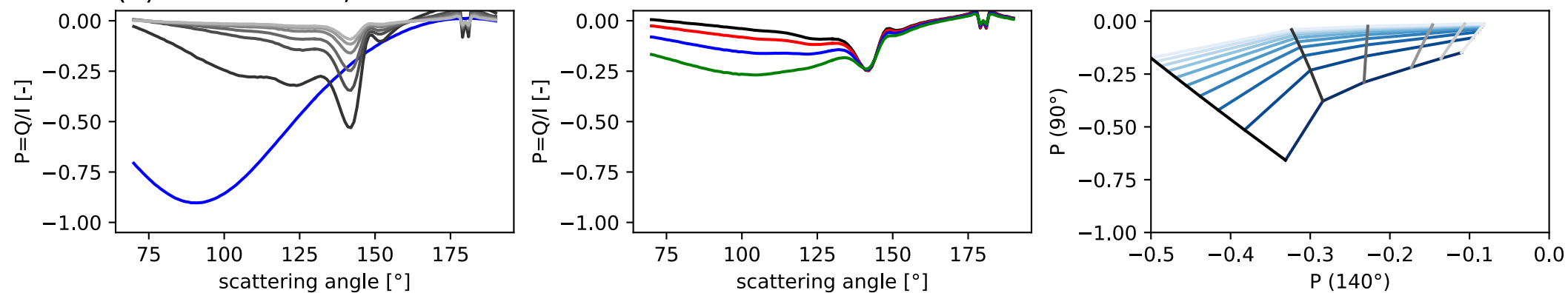
(d) dark surface, albedo = 0.0
