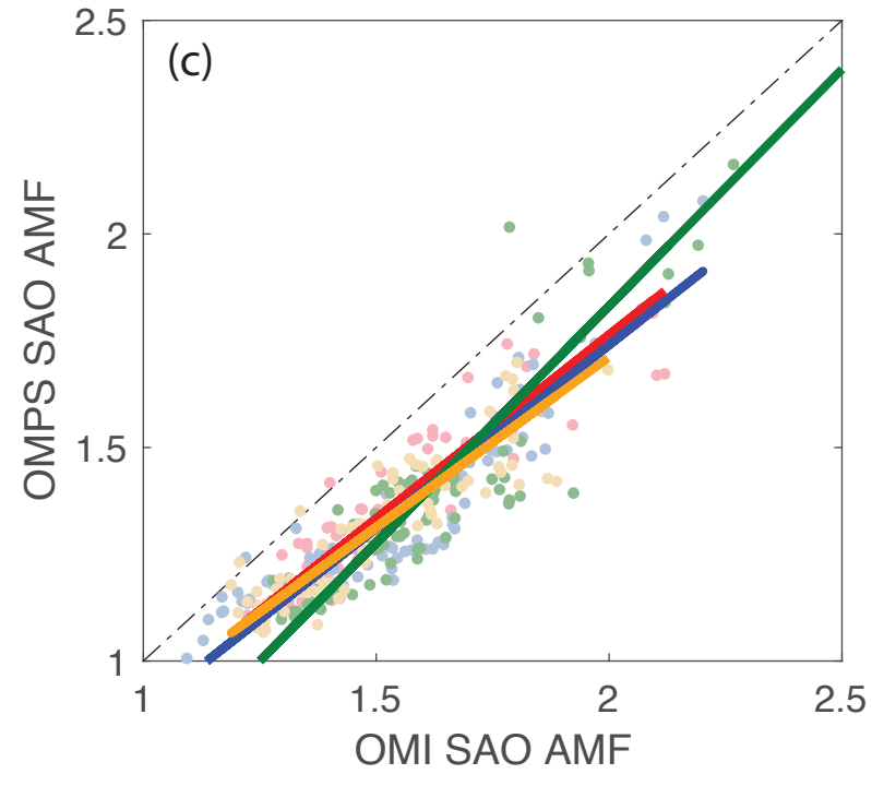
HCHO AMF
