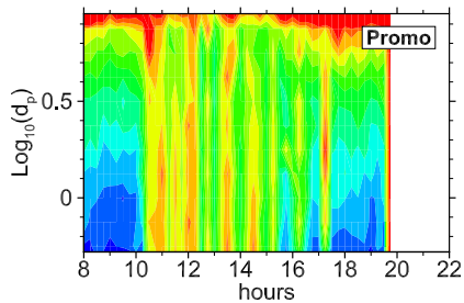
(b) Skewness
