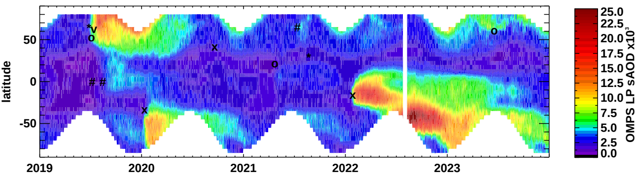
(b) sAOD (NRT) 997 nm
