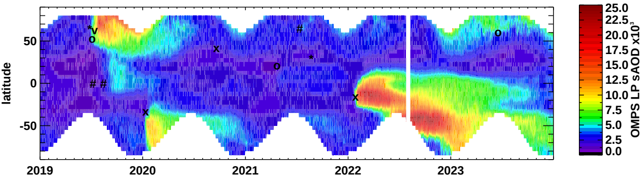
(b) sAOD (NRT) 997 nm
