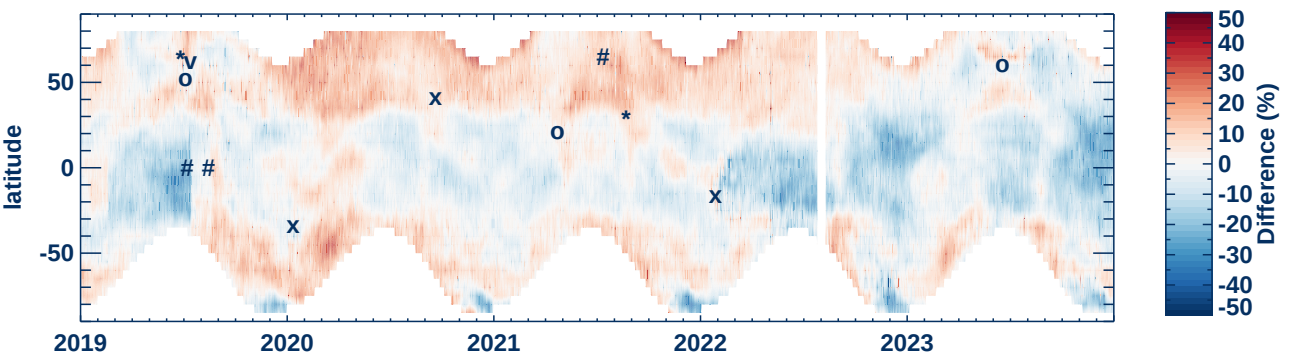
(c) sAOD NRT - V2.1 (%) 997 nm
