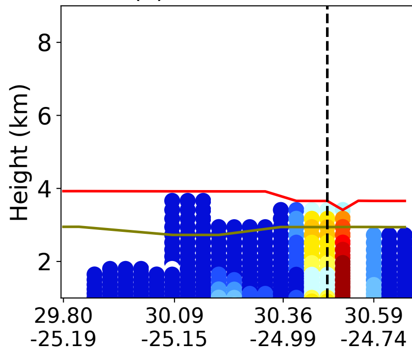
(d) Stratiform Rain
