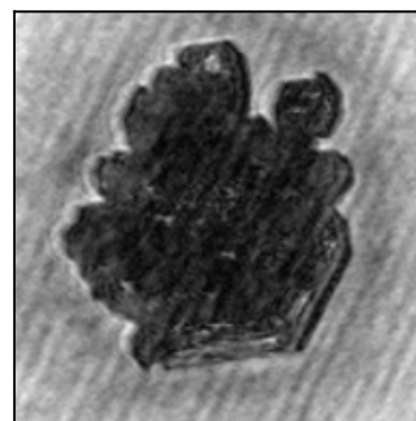
Plate_aged
