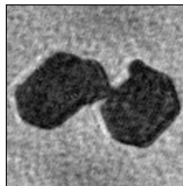
Plate_aged_aggregate
