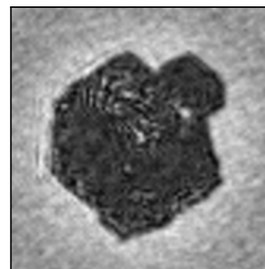
Plate_aggregate
