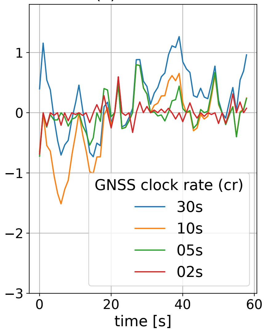
(d) BLOCK IIF
