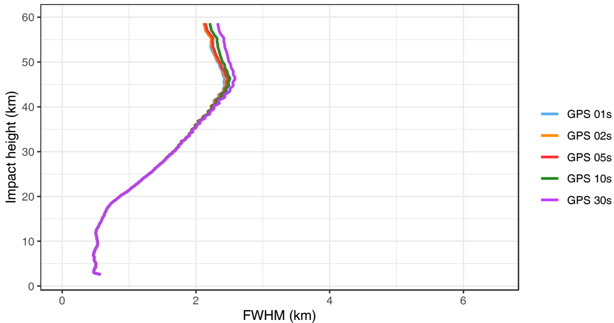
(b) S6A – GPS (GNSS: JPL dd s)
