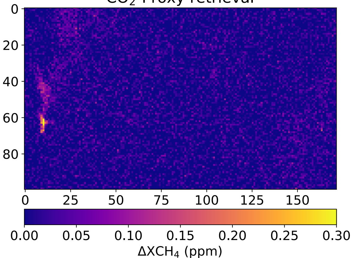
CO 2 -Proxy retrieval
