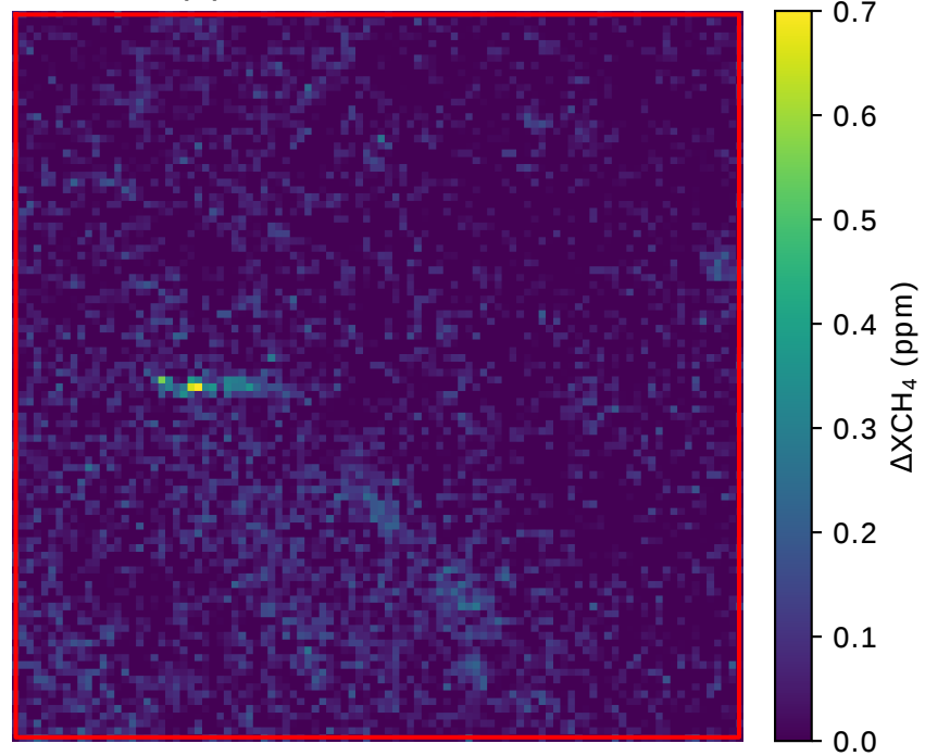
(d) EnMAP: 16/11/2022
