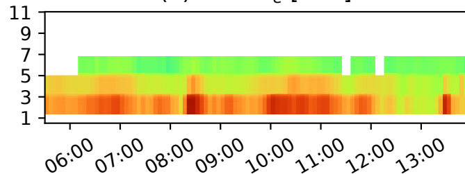
(d) MEM Z_e [dBZ]
