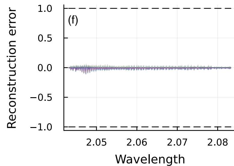
SCO2 Reconstruction + ILS
