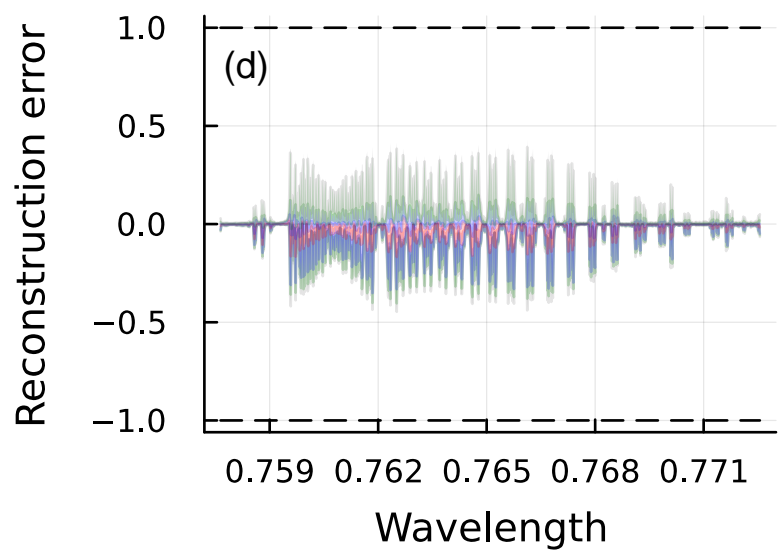
O2 Reconstruction + ILS
