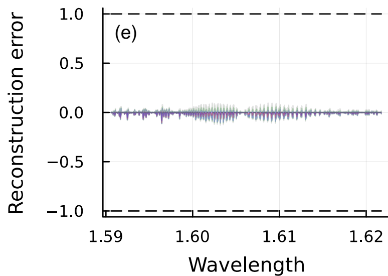
WCO2 Reconstruction + ILS
