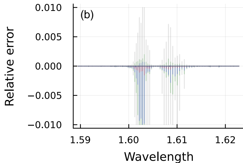
WCO2 Reconstruction
