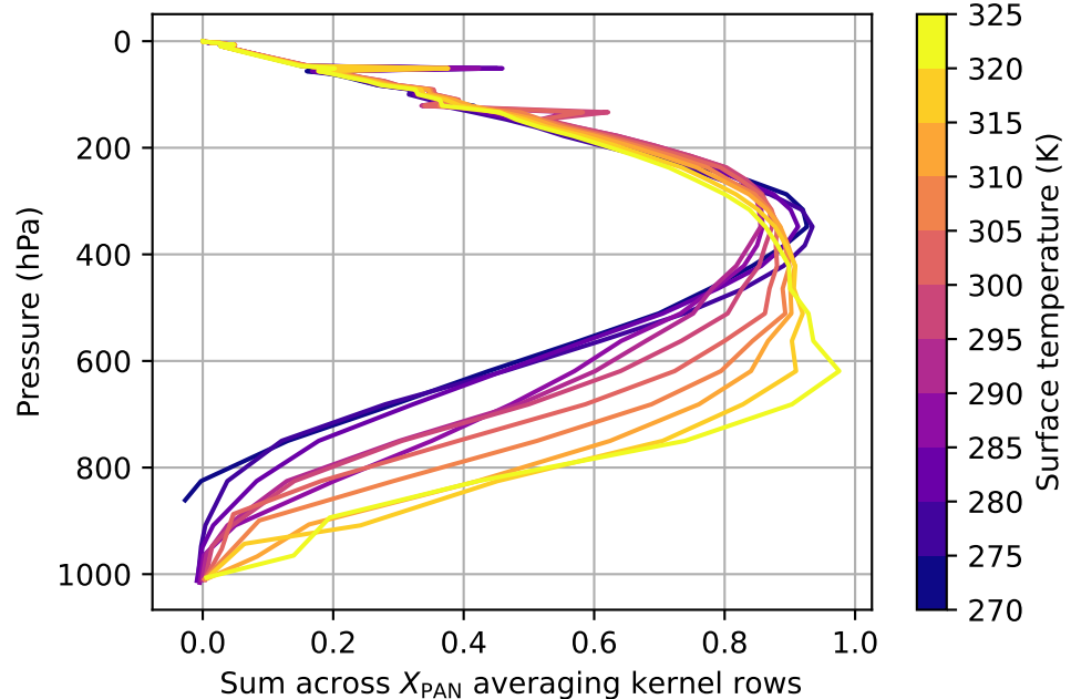
CrIS
