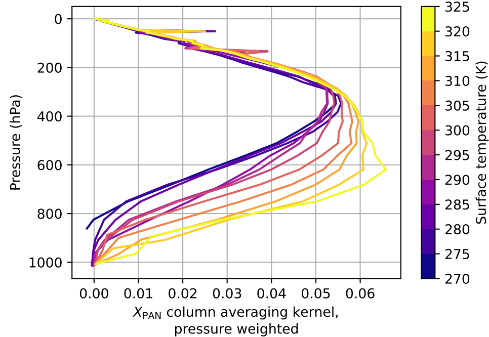
CrIS
