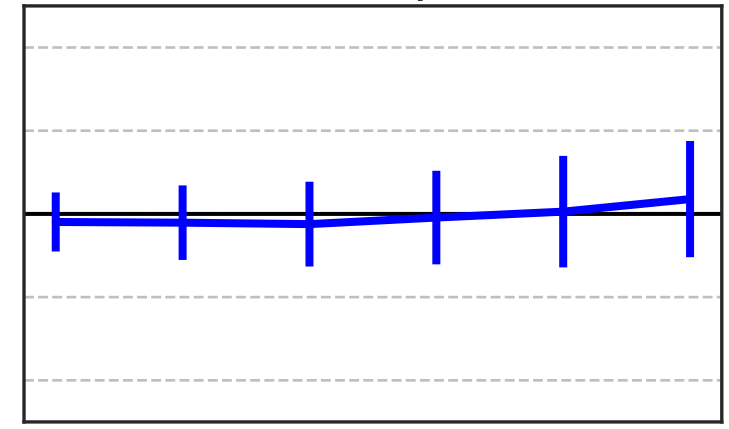
N. Hemisphere
