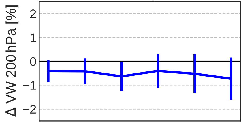
S. Hemisphere
