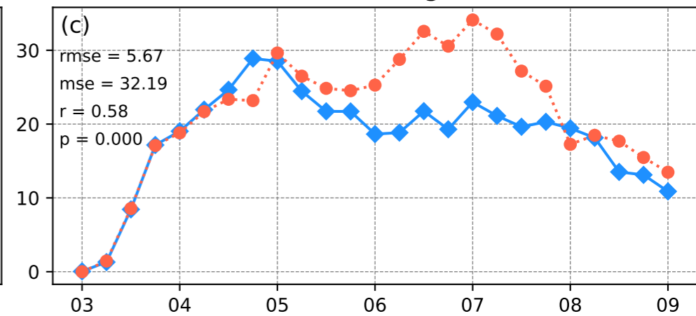
SO 2
