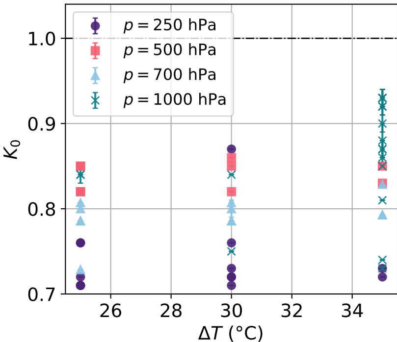
Butanol
