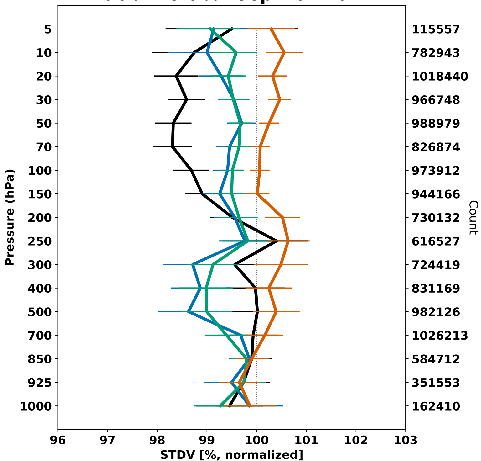
Raob-V Global Sep-Nov 2022
