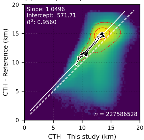
(d) SEVIRI, Mid-latitudes, 2004-2024
