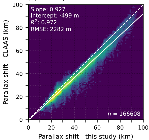
(d) Bias-adjusted to MODIS
