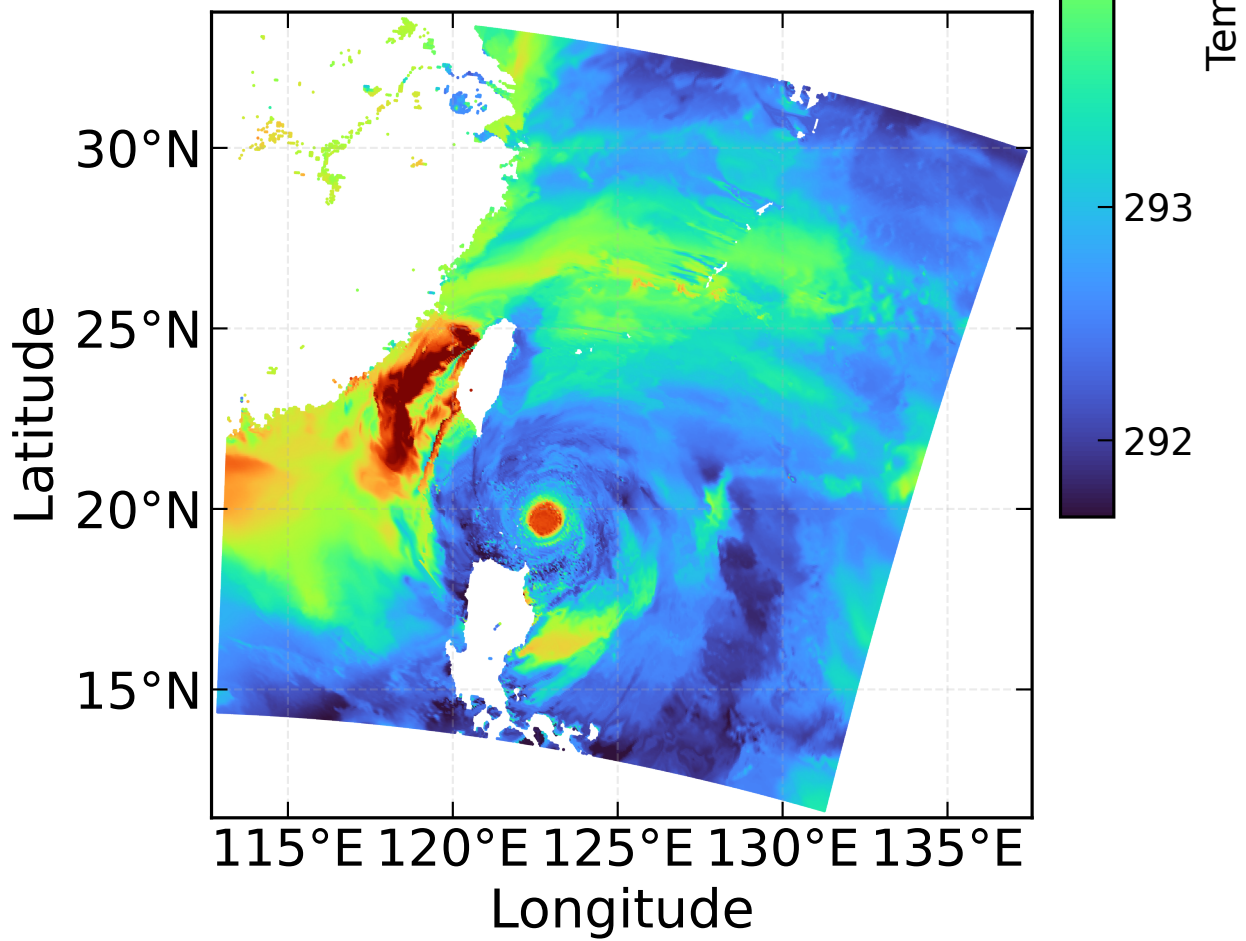
(d) Retrieval-850 hPa
