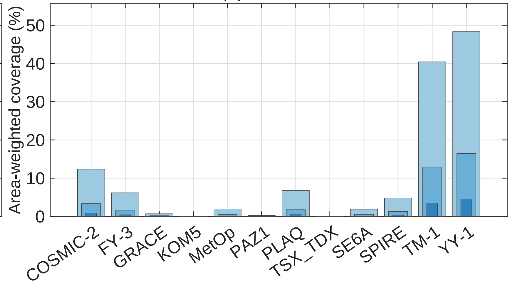
(d) 18–24 UTC
