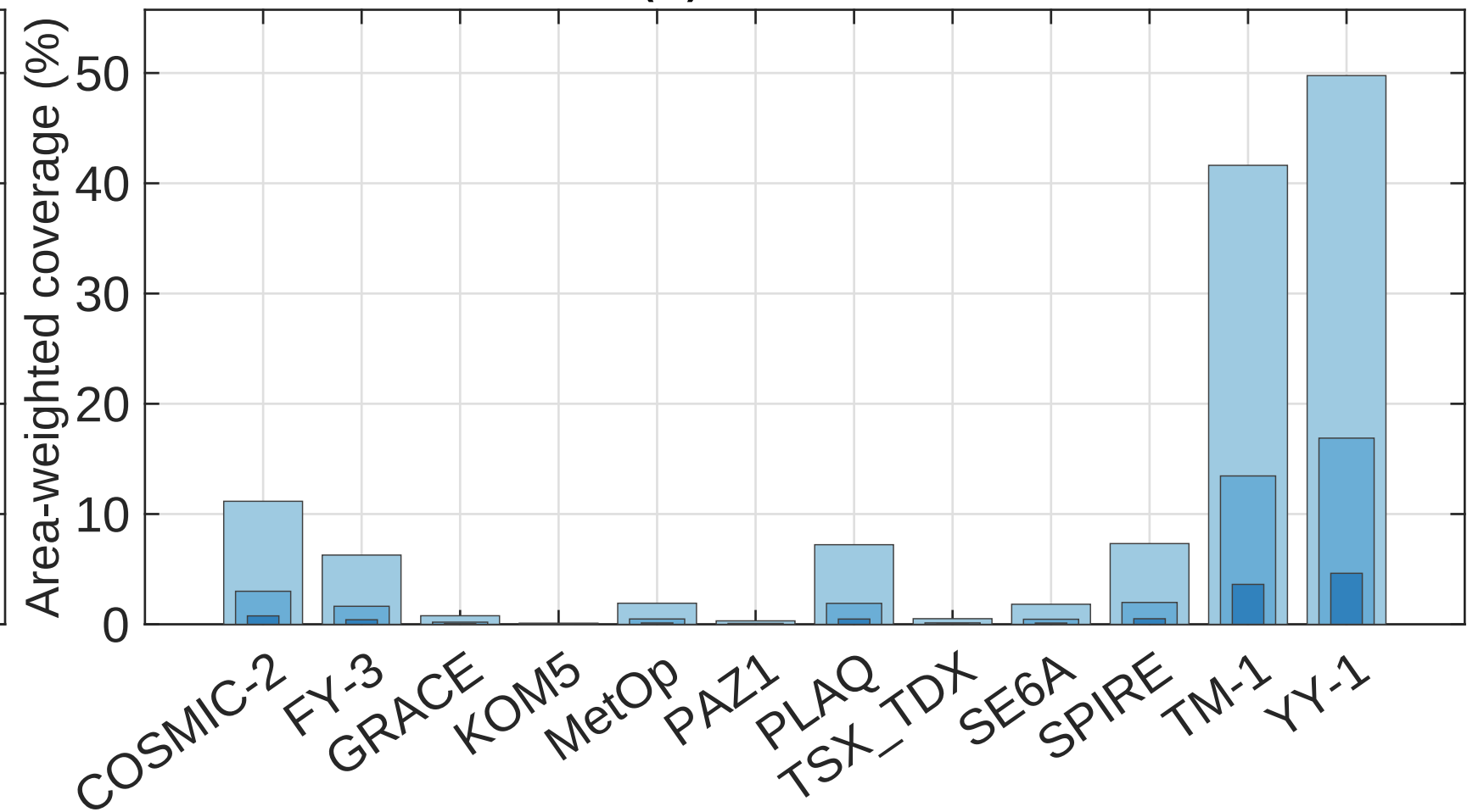
(d) 18–24 UTC
