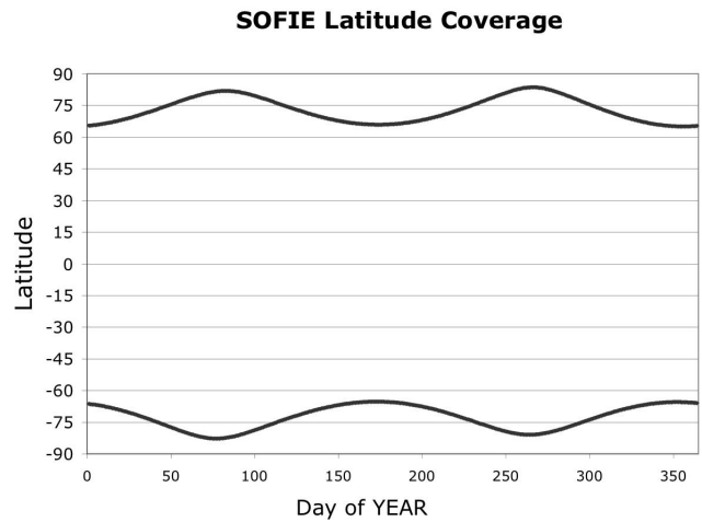
Fig. 29. SOFIE tangent-point latitudes.
