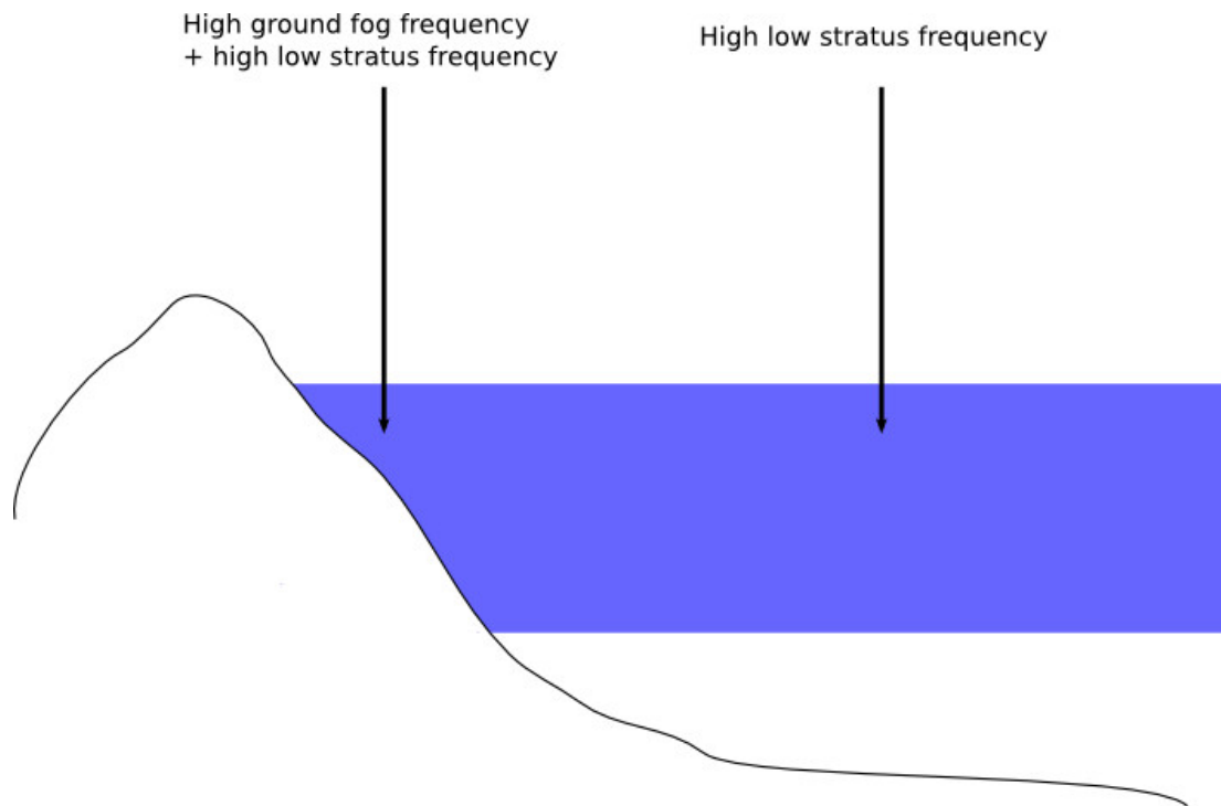
Fig. 1. fog vs. low stratus
